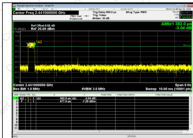
DH1
