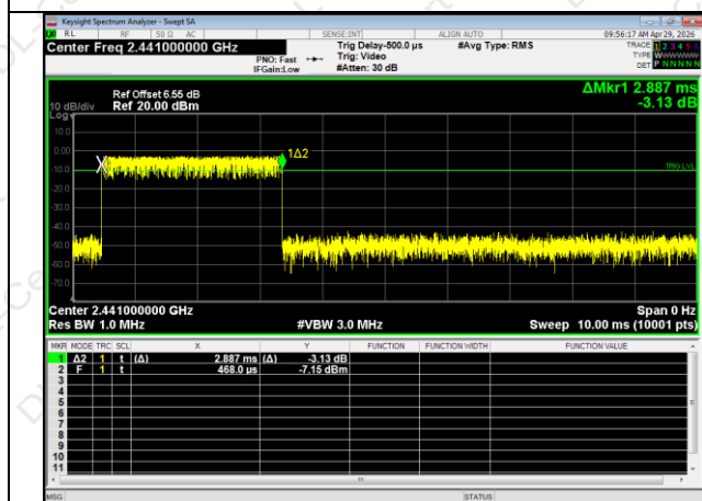
DH5
