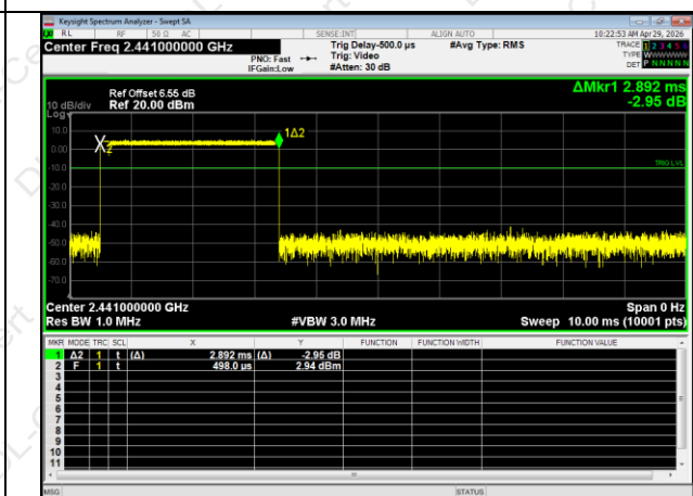
2-DH5
