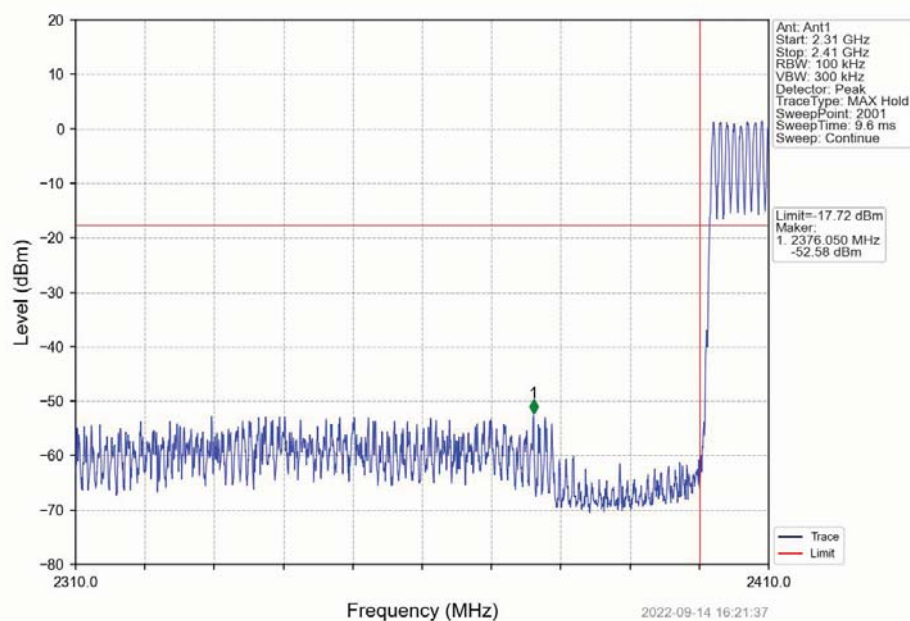
GFSK_DH5_HOPP_2410MHz_Ant1_NTNV
