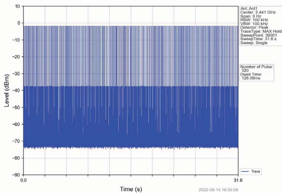
8DPSK_3DH1_HOPP_Ant1_NTNV
