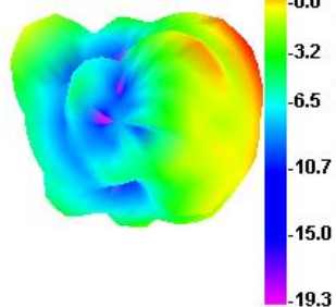
2450.000MHz
