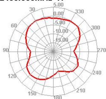
2450.000MHz H
