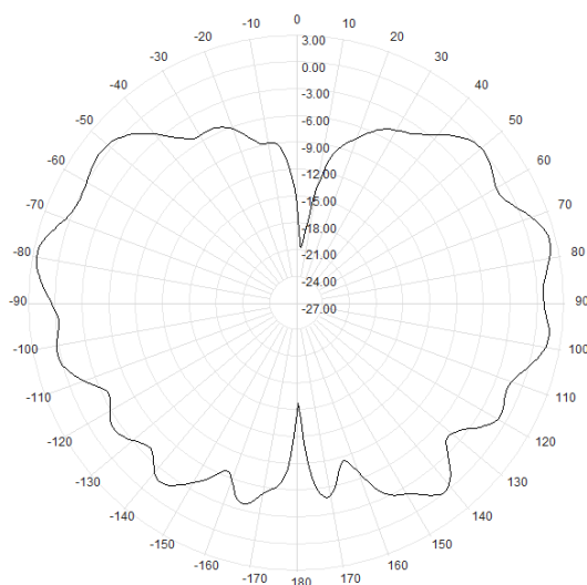
E(930MHz)
