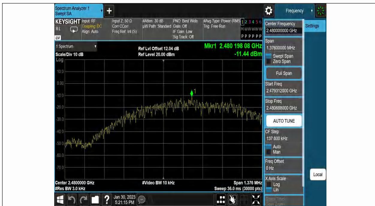
BLE 1M-Ant1-2480--11.44-0.00-0.00-0.00
