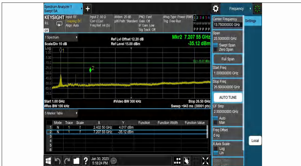
BLE 1M-Ant1-2402-1000~26500-4.39
