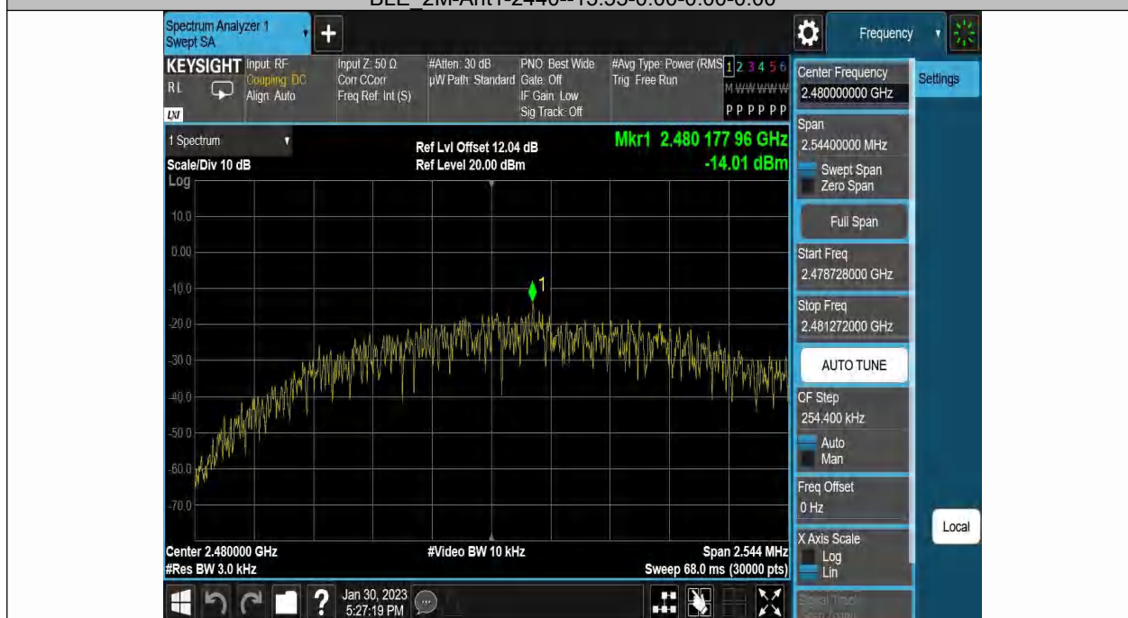
BLE 2M-Ant1-2480--14.01-0.00-0.00-0.00
