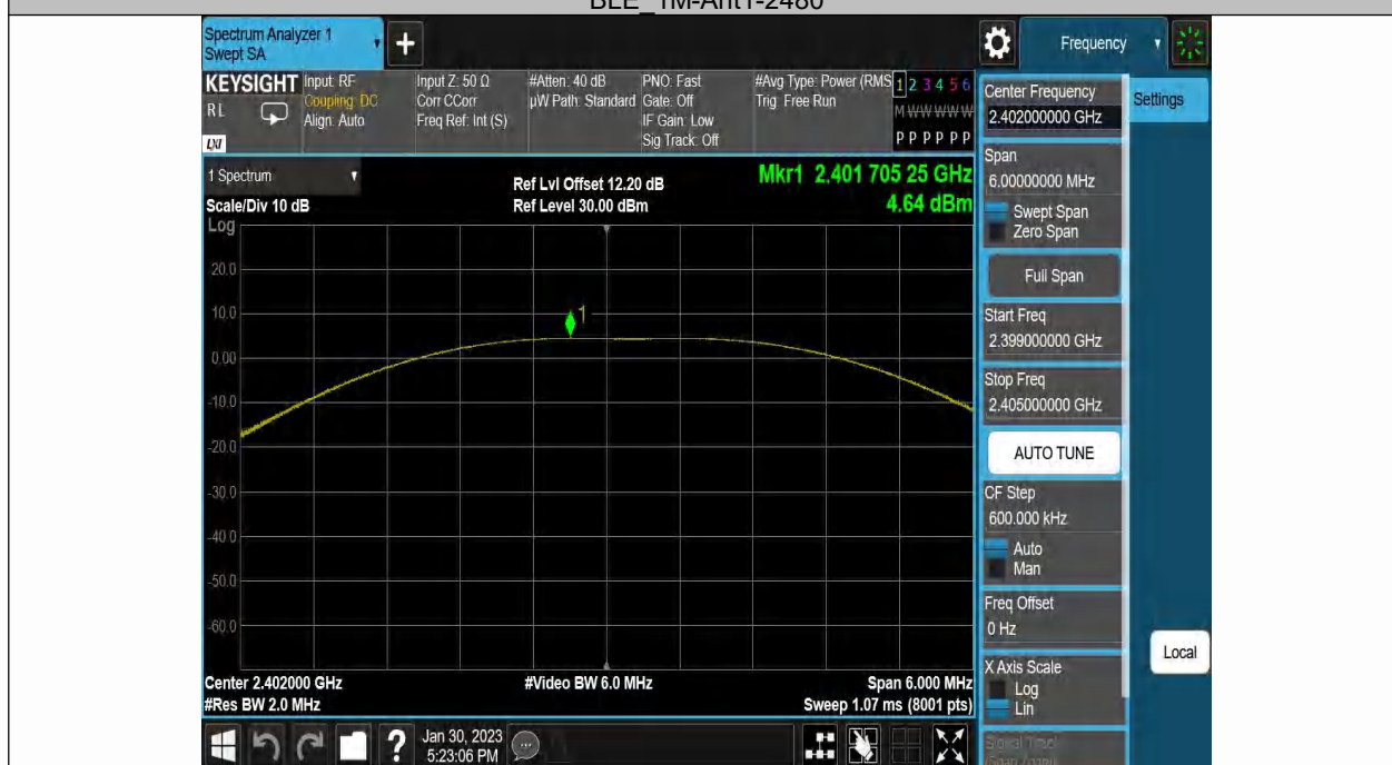
BLE_2M-Ant1-2402
