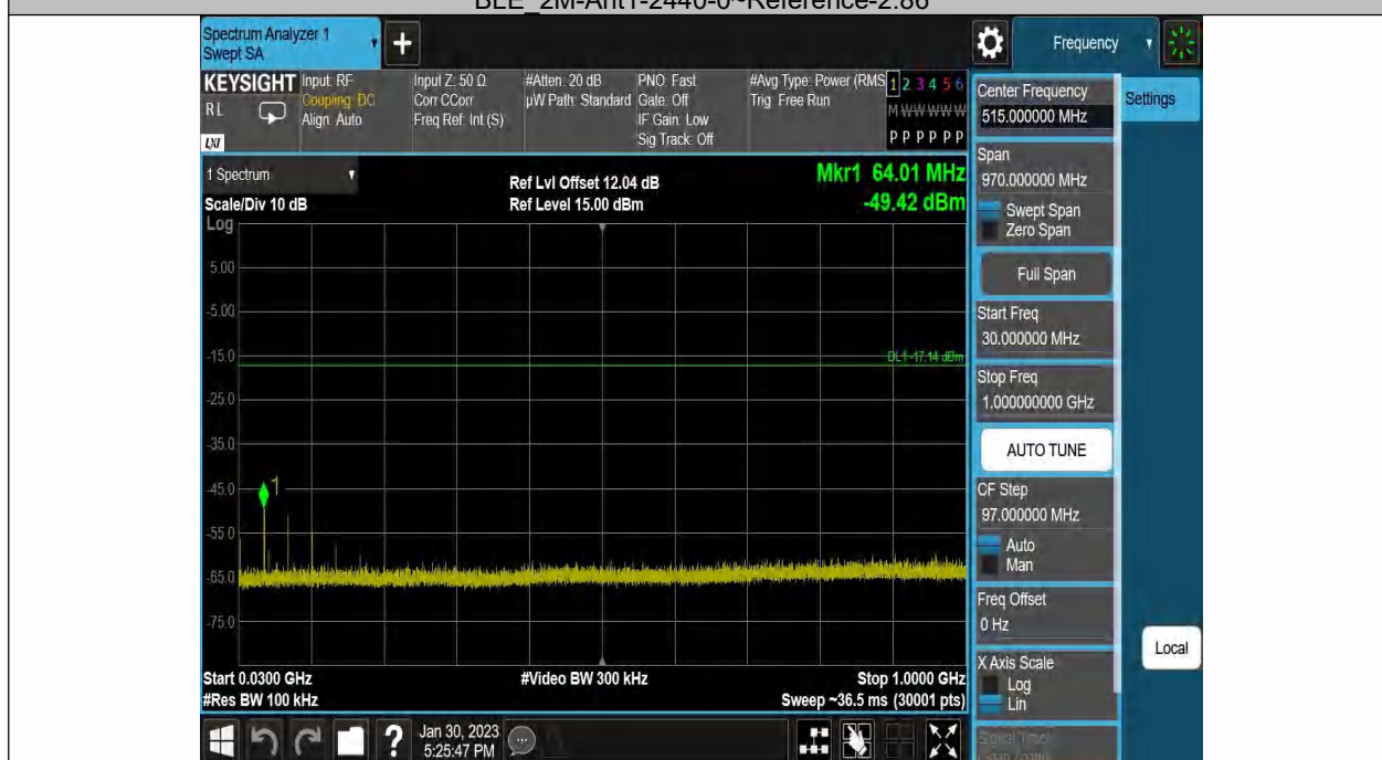
BLE_2M-Ant1-2440-30~1000-2.86
