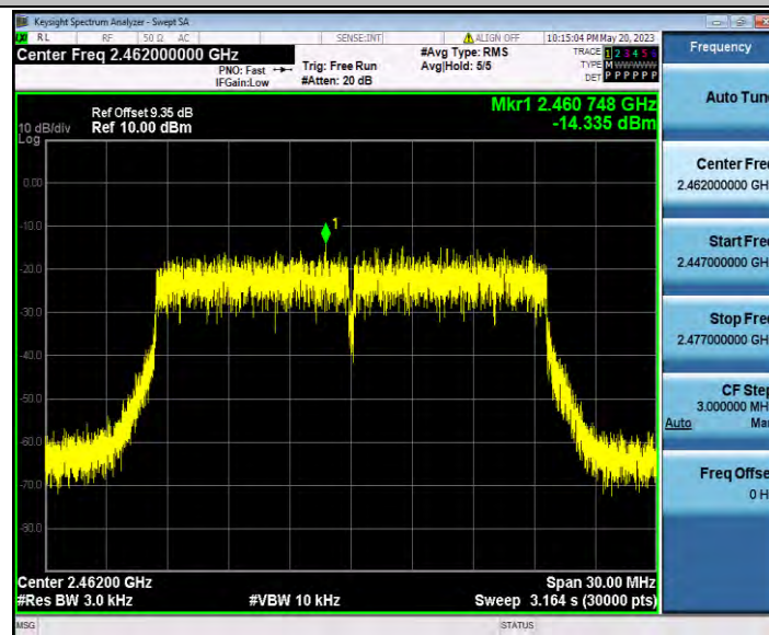
11AX20SISO_Ant2_2462
