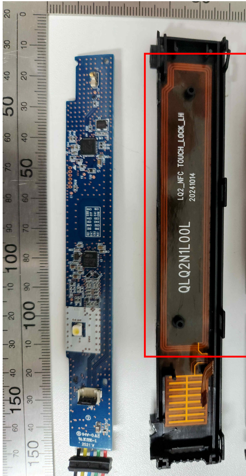
Antenna
