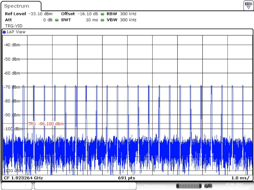
35 µs Pulses
