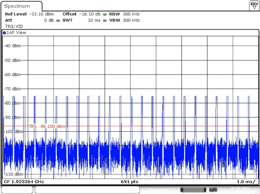
50 µs Pulses
