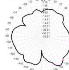
2500.0MHz Total(E2-YZ), Max= 5.39dBi
