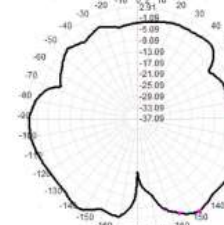
2400.0MHz Total(E2-YZ), Max= 2.91dBi
