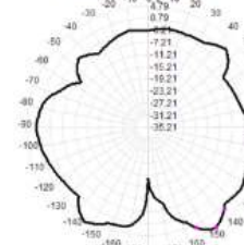
2450.0MHz Total(E2-YZ), Max= 4.79dBi
