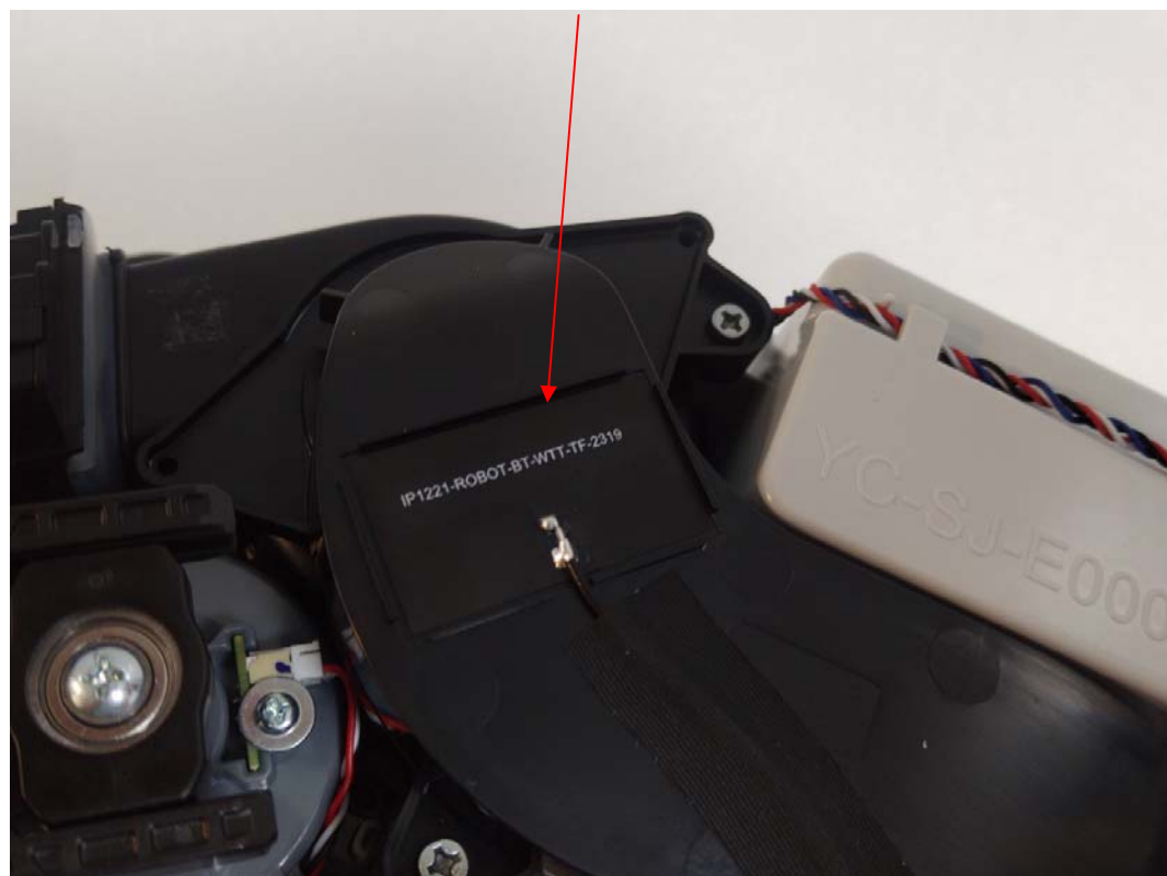
BLE Antenna
