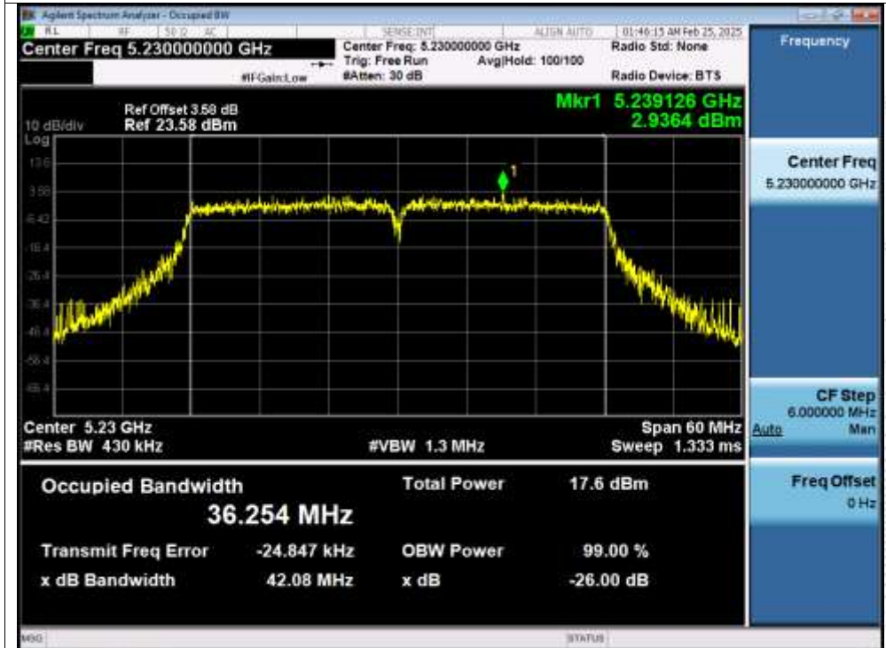
-26dB Bandwidth NVNT n40 5230MHz
