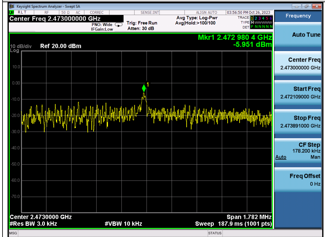
Test_Graph_GFSK_ANT1_2473_PSD
