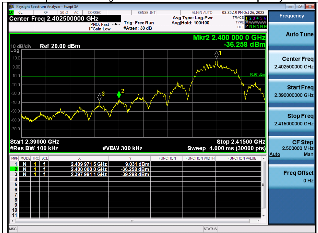
Test_Graph_GFSK_ANT1_2410_Lower Band Edge Emissions
