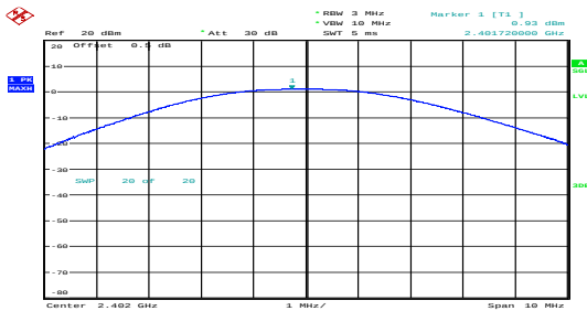
Low 0.93dBm
