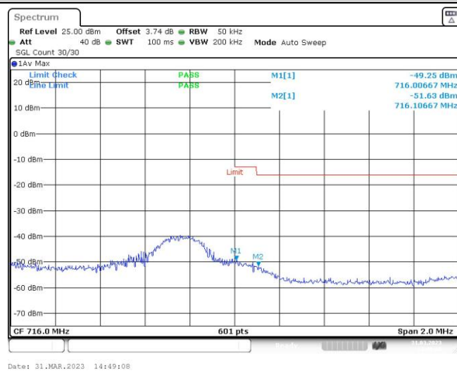
Band12-3MHz-QPSK-23165-1RB#14
