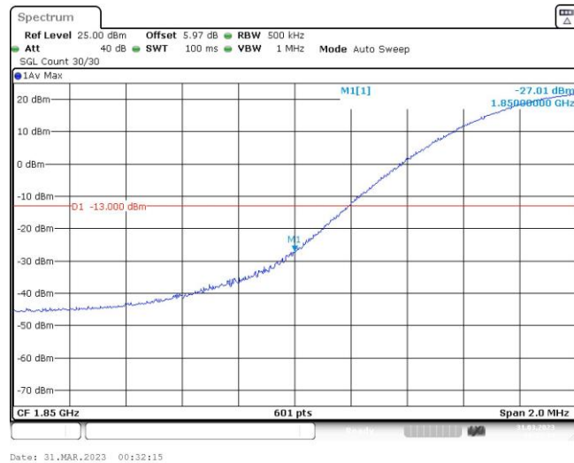
Band2-20MHz-QPSK-18700-1RB#99
