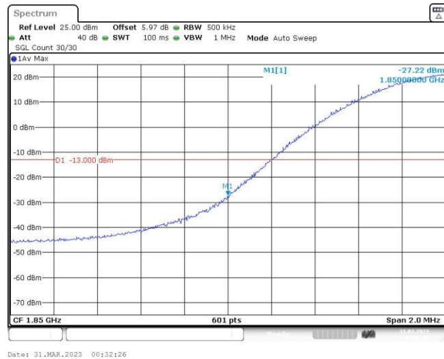
Band2-20MHz-16QAM-18700-1RB#99
