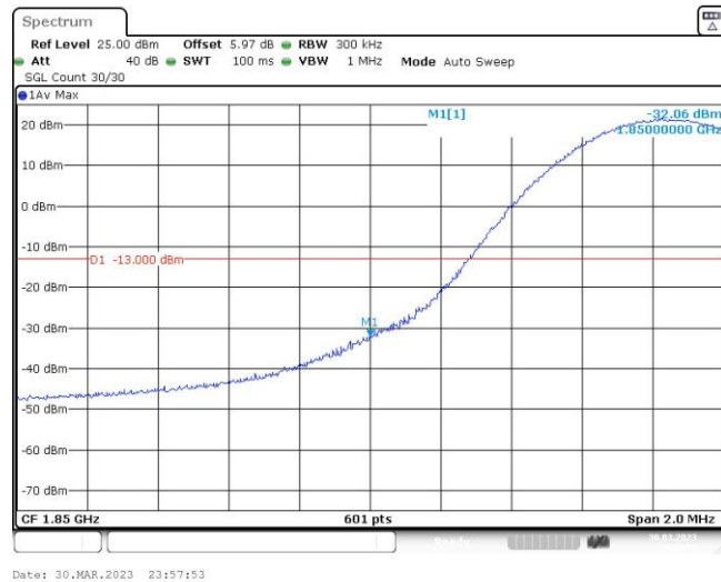
Band2-15MHz-16QAM-18675-1RB#74
