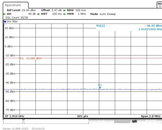
Band25-20MHz-QPSK-26590-1RB#99
