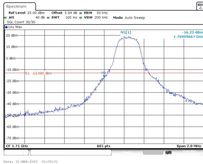
Band4-3MHz-QPSK-19965-1RB#14
