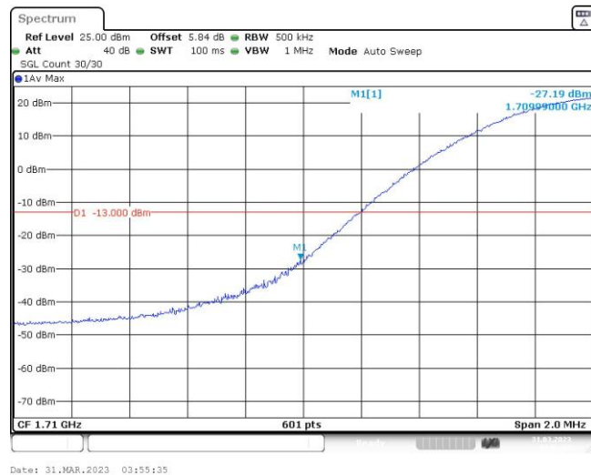
Band4-20MHz-QPSK-20050-1RB#99
