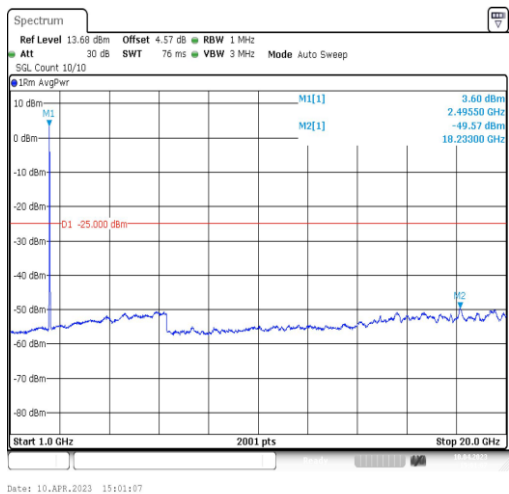
41-41-5MHz-20MHz-QPSK-QPSK-39683-39800-25RB#0-100RB#0-1000~20000MHz
