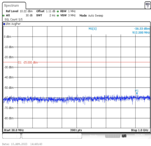
41-41-5MHz-20MHz-QPSK-QPSK-39683-39800-1RB#0-0RB#0-30~1000MHz
