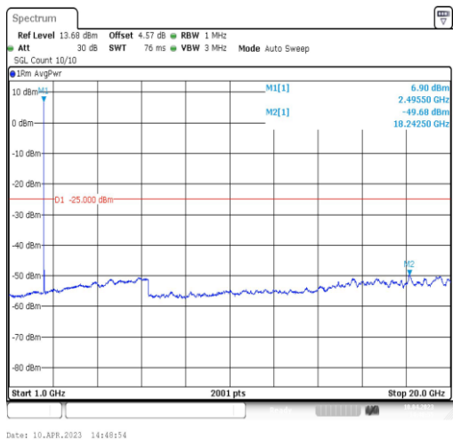
41-41-5MHz-20MHz-QPSK-QPSK-39683-39800-1RB#0-0RB#0-1000~20000MHz
