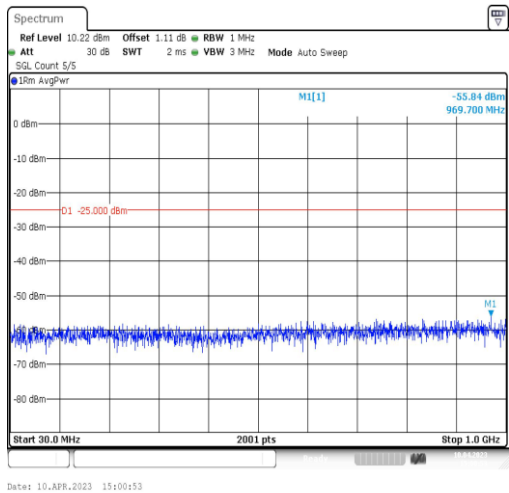
41-41-5MHz-20MHz-QPSK-QPSK-39683-39800-25RB#0-100RB#0-30~1000MHz
