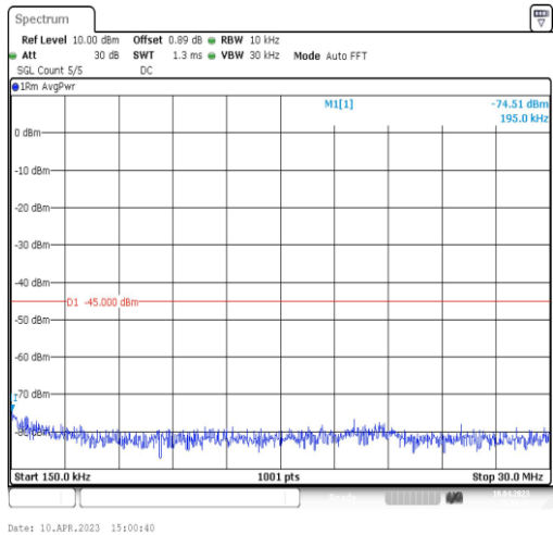
41-41-5MHz-20MHz-QPSK-QPSK-39683-39800-25RB#0-100RB#0-0.15~30MHz
