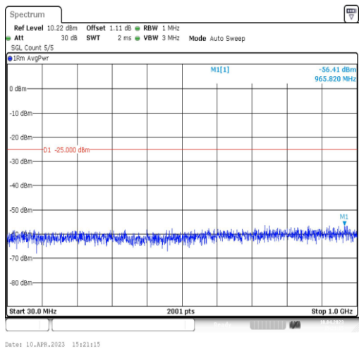
41-41-5MHz-20MHz-QPSK-QPSK-41373-41490-1RB#0-0RB#0-30~1000MHz
