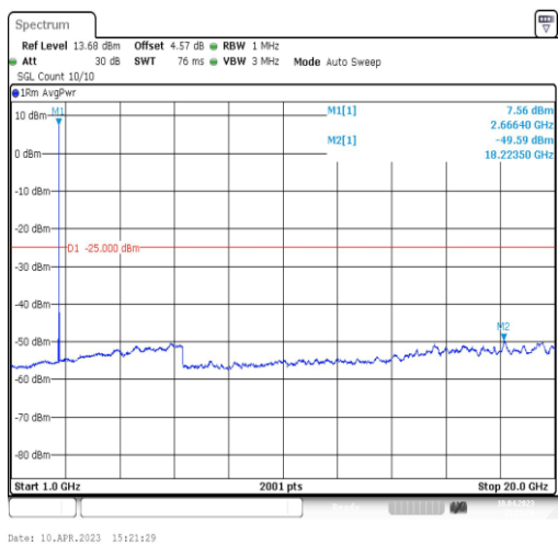
41-41-5MHz-20MHz-QPSK-QPSK-41373-41490-1RB#0-0RB#0-1000~20000MHz
