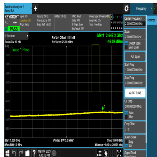
NTNV_N41_PC2_30_40_L_TID4_N/A_1000_300 0_#1
