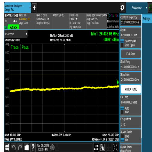
NTNV_N41_PC2_30_20_M_TID5_N/A_18000_26500_#1
