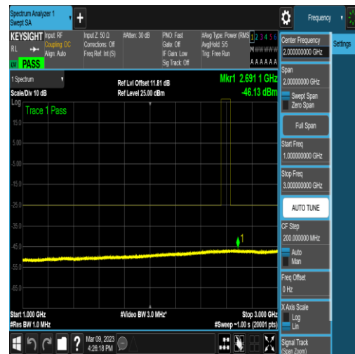
NTNV_N41_PC2_30_20_M_TID17_N/A_1000_30 00_#1
