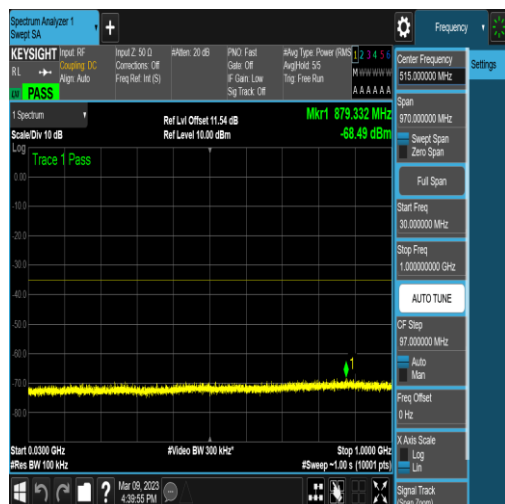
NTNV_N41_PC2_30_40_L_TID4_N/A_30_1000_#1
