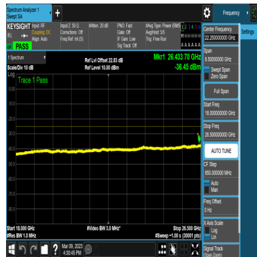
NTNV_N41_PC2_30_20_H_TID4_N/A_18000_26500_#1
