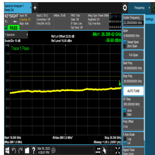
NTNV_N41_PC2_30_20_H_TID18_N/A_18000_2 6500_#1
