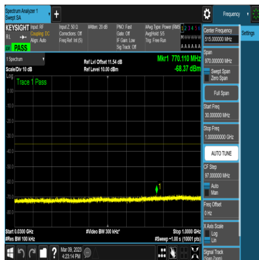
NTNV_N41_PC2_30_20_M_TID6_N/A_30_1000_#1
