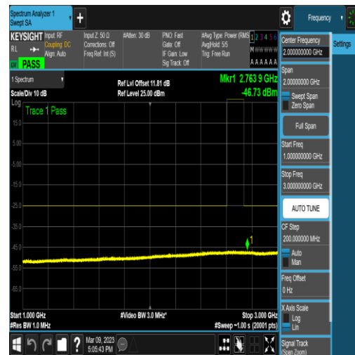
NTNV_N41_PC2_30_40_H_TID4_N/A_1000_300 0_#1
