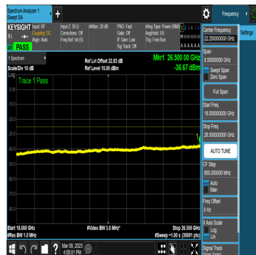
NTNV_N41_PC2_30_40_M_TID5_N/A_18000_26 500_#1
