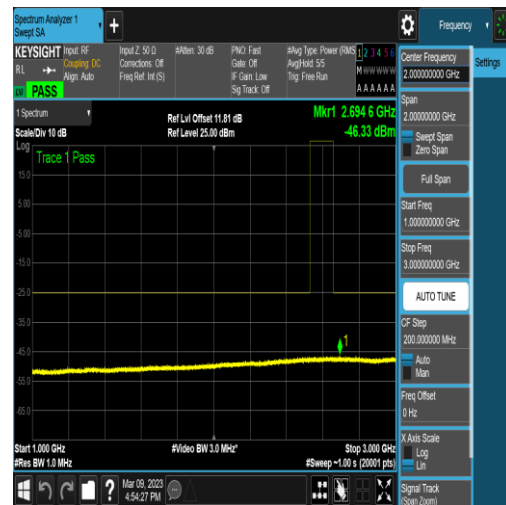
NTNV_N41_PC2_30_40_M_TID5_N/A_1000_300 0_#1
