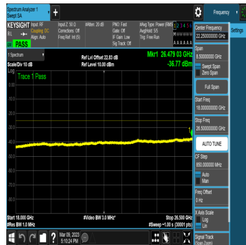
NTNV_N41_PC2_30_40_H_TID6_N/A_18000_26500_#1
