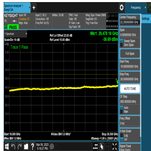
NTNV_N41_PC2_30_60_L_TID5_N/A_18000_26500_#1
