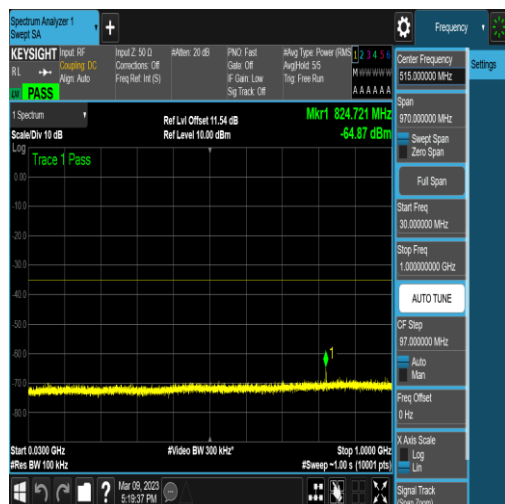
NTNV_N41_PC2_30_60_L_TID6_N/A_30_1000_#1
