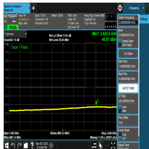
NTNV_N41_PC2_30_60_L_TID6_N/A_1000_300_0_#1
