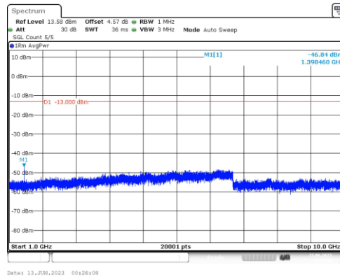
Band12-1.4MHz-QPSK-23017-1RB#0-Range4:1000~10000MHz
