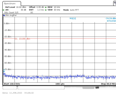
Band12-1.4MHz-16QAM-23017-1RB#0-Range2:0.15~30MHz
