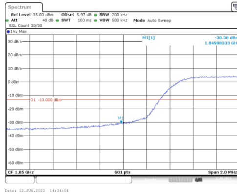
Band2-10MHz-QPSK-18650-50RB#0
