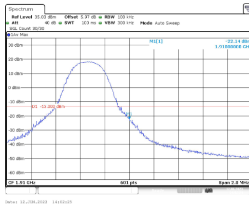
Band2-5MHz-QPSK-19175-1RB#24
