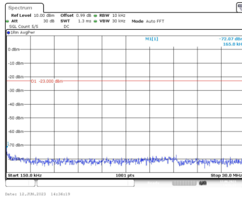
Band2-10MHz-QPSK-18650-1RB#0-Range2:0.15~30MHz
