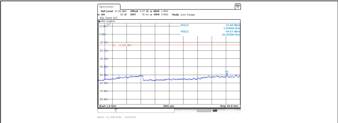
Band2-5MHz-QPSK-18900-1RB#0-Range4:1000~20000MHz
