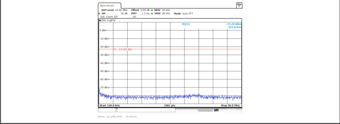
Band2-10MHz-QPSK-19150-1RB#0-Range2:0.15~30MHz
