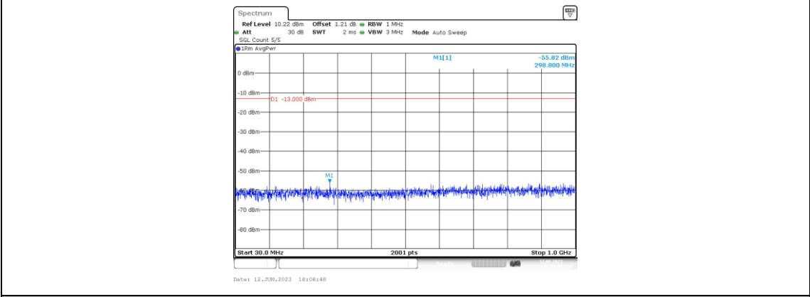
Band2-20MHz-QPSK-19100-1RB#0-Range3:30~1000MHz
