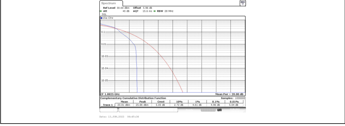
Band25-10MHz-QPSK-26365-1RB#0
