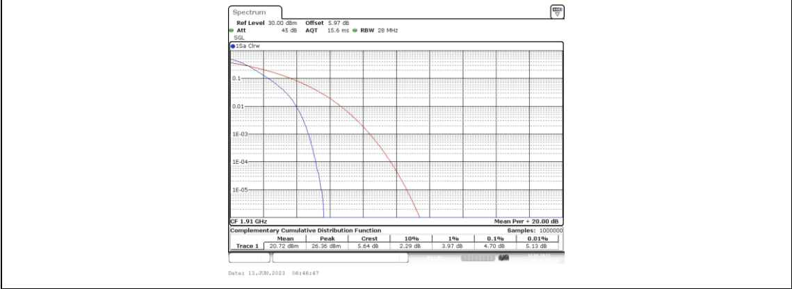
Band25-10MHz-QPSK-26640-50RB#0
