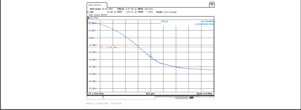
Band25-20MHz-QPSK-26590-1RB#99
