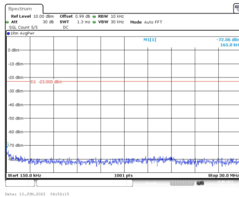
Band25-1.4MHz-QPSK-26683-1RB#0-Range2:0.15~30MHz
