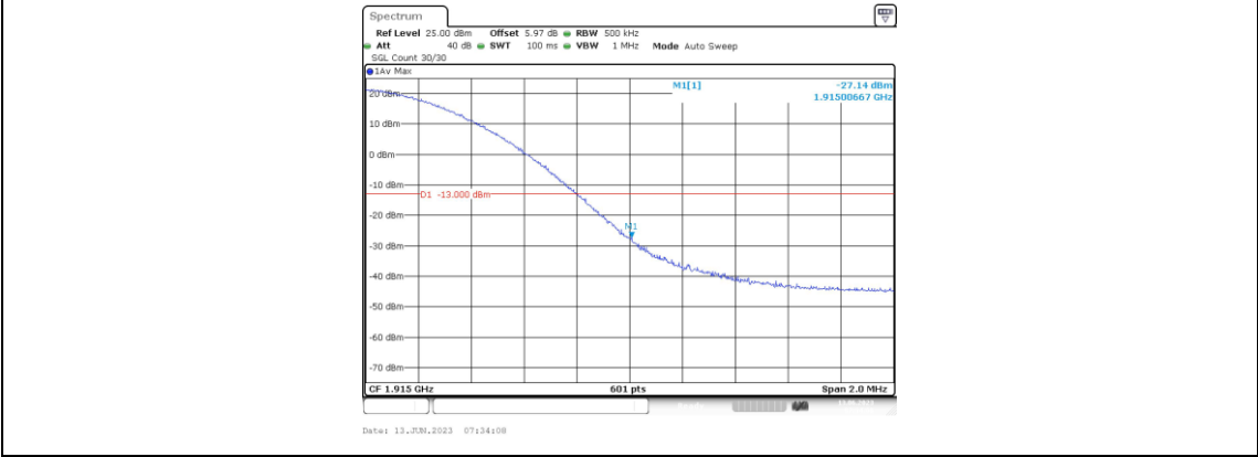
Band25-20MHz-QPSK-26590-1RB#99
