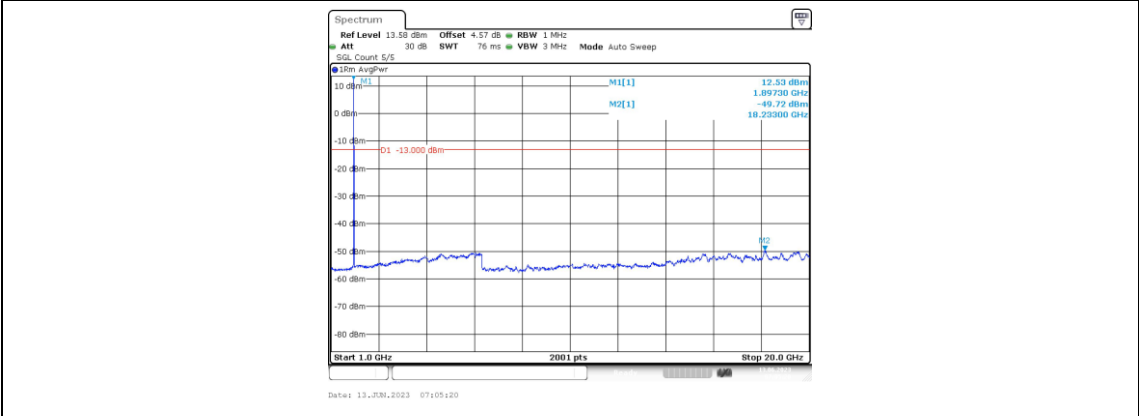
Band25-15MHz-QPSK-26615-1RB#0-Range4:1000~20000MHz
