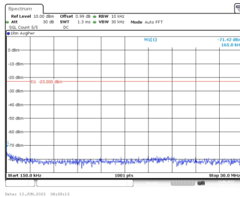
Band25-10MHz-QPSK-26090-1RB#0-Range2:0.15~30MHz
