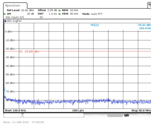
Band25-20MHz-QPSK-26365-1RB#0-Range2:0.15~30MHz
