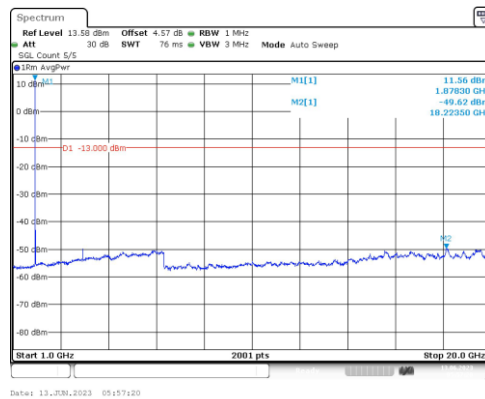
Band25-5MHz-QPSK-26365-1RB#0-Range4:1000~20000MHz
