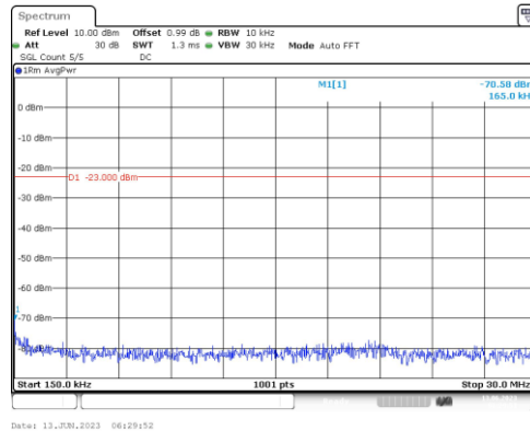
Band25-10MHz-QPSK-26365-1RB#0-Range2:0.15~30MHz
