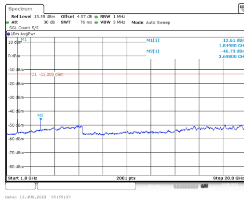
Band25-5MHz-QPSK-26065-1RB#0-Range4:1000~20000MHz
