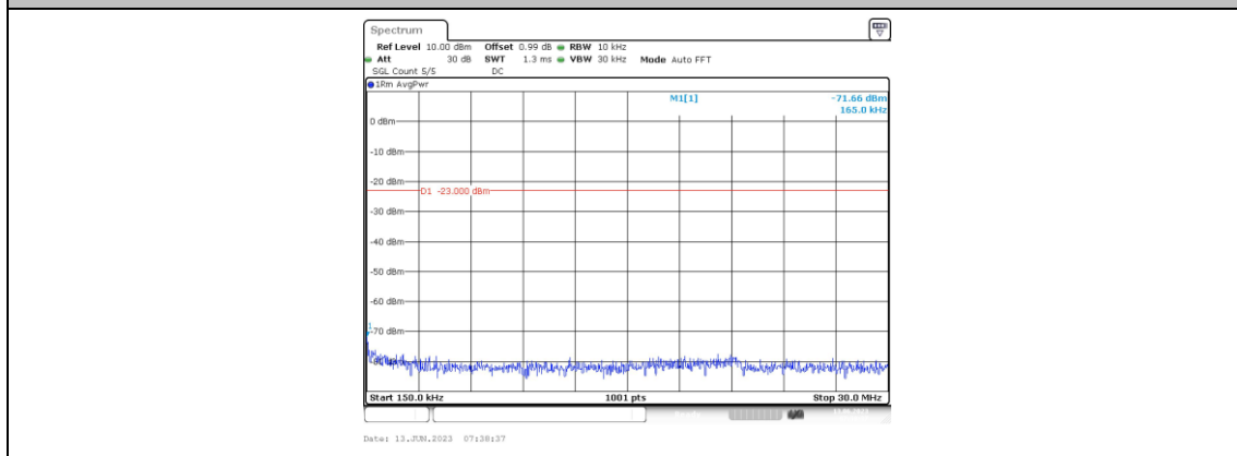
Band25-20MHz-QPSK-26590-1RB#0-Range2:0.15~30MHz
