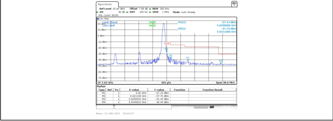
Band38-15MHz-QPSK-38175-1RB#74
