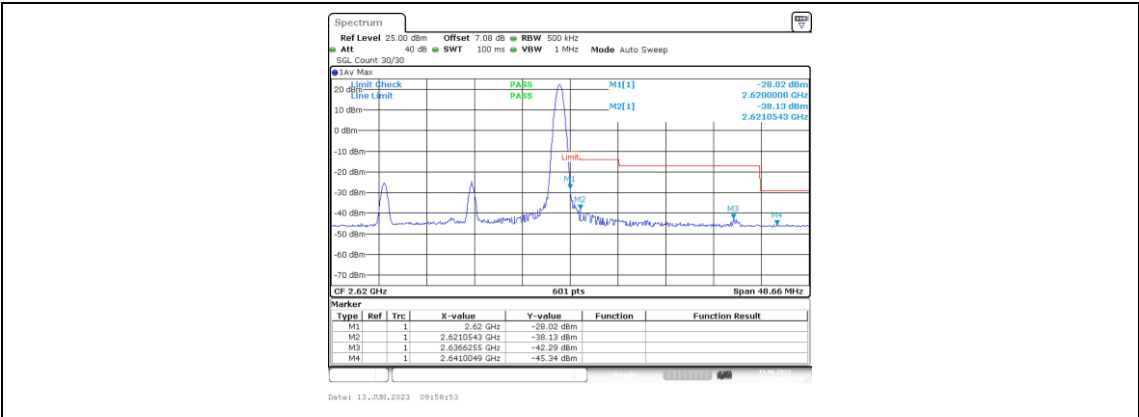
Band38-20MHz-QPSK-38150-1RB#99
