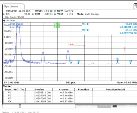
Band38-20MHz-QPSK-38150-1RB#0
