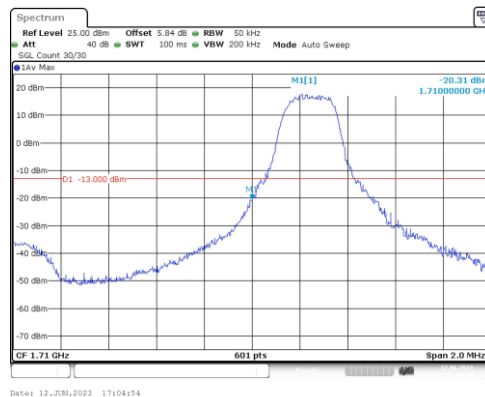
Band4-3MHz-QPSK-19965-1RB#0
