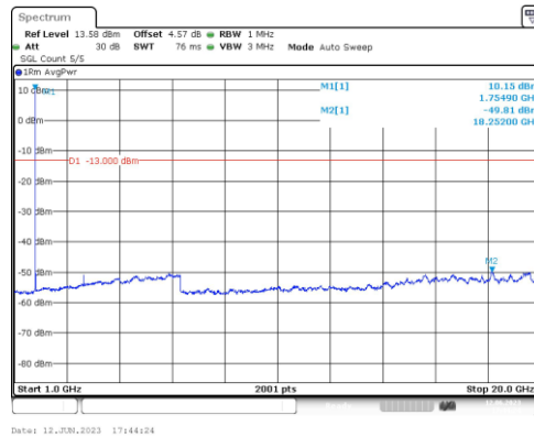
Band4-5MHz-QPSK-20375-1RB#0-Range4:1000~20000MHz
