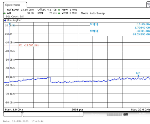
Band4-5MHz-QPSK-20175-1RB#0-Range4:1000~20000MHz
