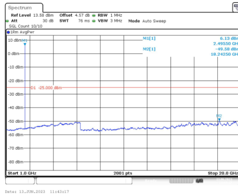
Band41-5MHz-QPSK-39675-1RB#0-Range4:1000~20000MHz
