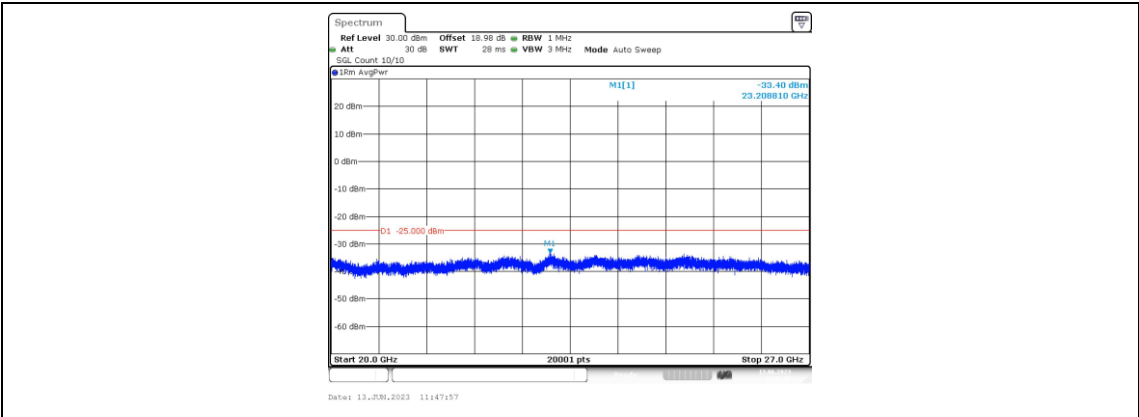
Band41-5MHz-QPSK-41565-1RB#0-Range5:20000~27000MHz
