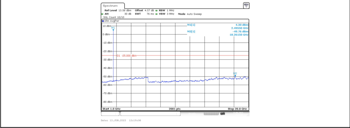
Band41-10MHz-QPSK-39700-1RB#0-Range4:1000~20000MHz
