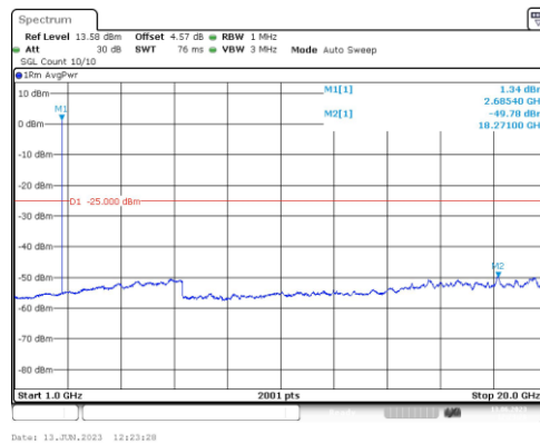
Band41-10MHz-QPSK-41540-1RB#0-Range4:1000~20000MHz
