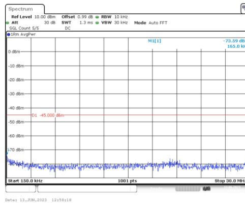
Band41-15MHz-QPSK-41515-1RB#0-Range2:0.15~30MHz
