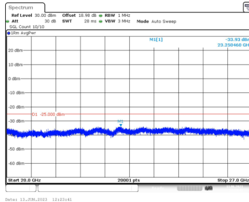
Band41-10MHz-QPSK-41540-1RB#0-Range5:20000~27000MHz
