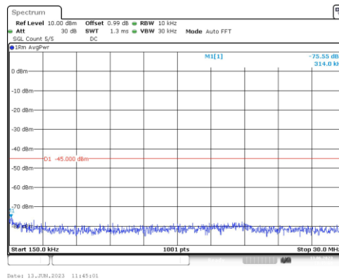
Band41-5MHz-QPSK-40620-1RB#0-Range2:0.15~30MHz
