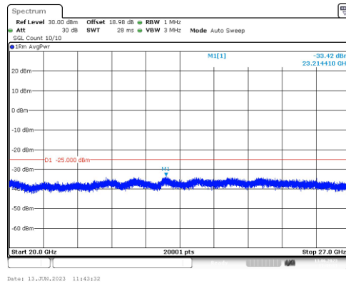
Band41-5MHz-QPSK-39675-1RB#0-Range5:20000~27000MHz
