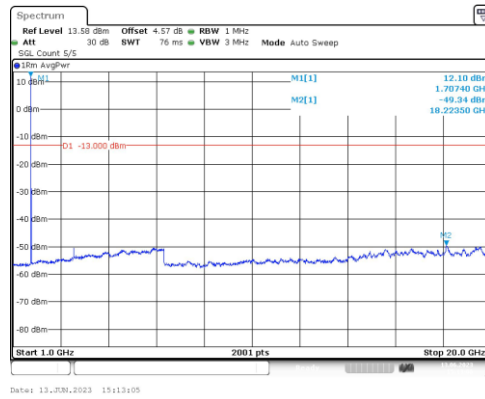
Band66-5MHz-QPSK-131997-1RB#0-Range4:1000~20000MHz
