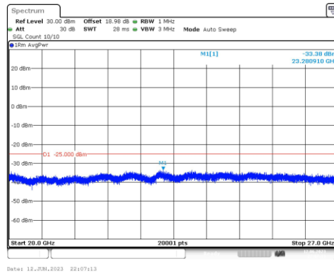
Band7-5MHz-QPSK-20775-1RB#0-Range5:20000~27000MHz
