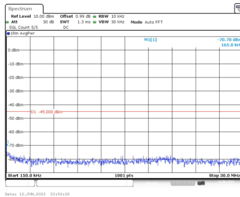
Band7-20MHz-QPSK-21100-1RB#0-Range2:0.15~30MHz
