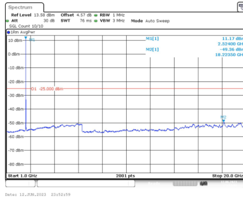
Band7-20MHz-QPSK-21100-1RB#0-Range4:1000~20000MHz
