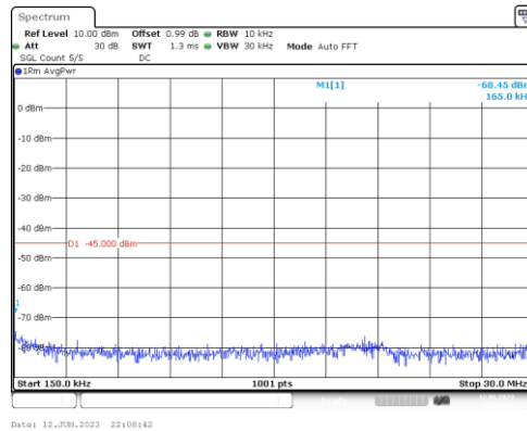
Band7-5MHz-QPSK-21100-1RB#0-Range2:0.15~30MHz
