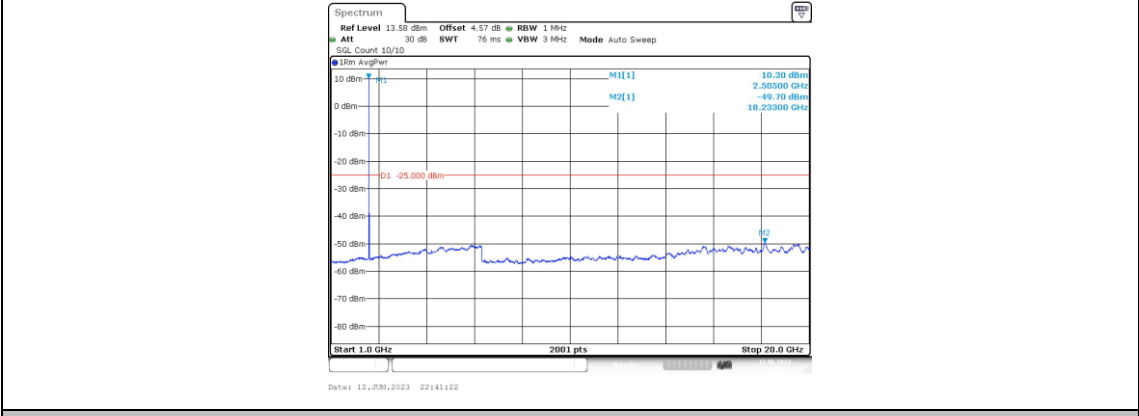
Band7-10MHz-QPSK-20800-1RB#0-Range4:1000~20000MHz
