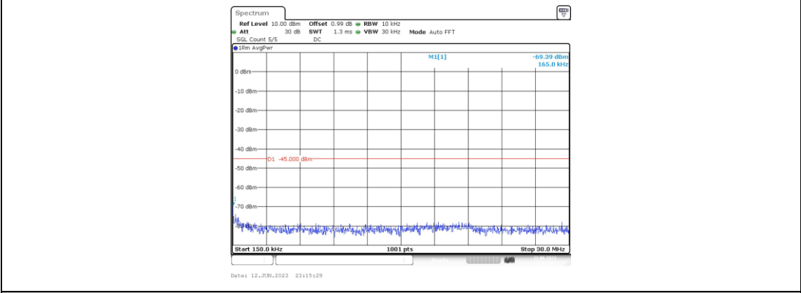
Band7-15MHz-QPSK-20825-1RB#0-Range2:0.15~30MHz
