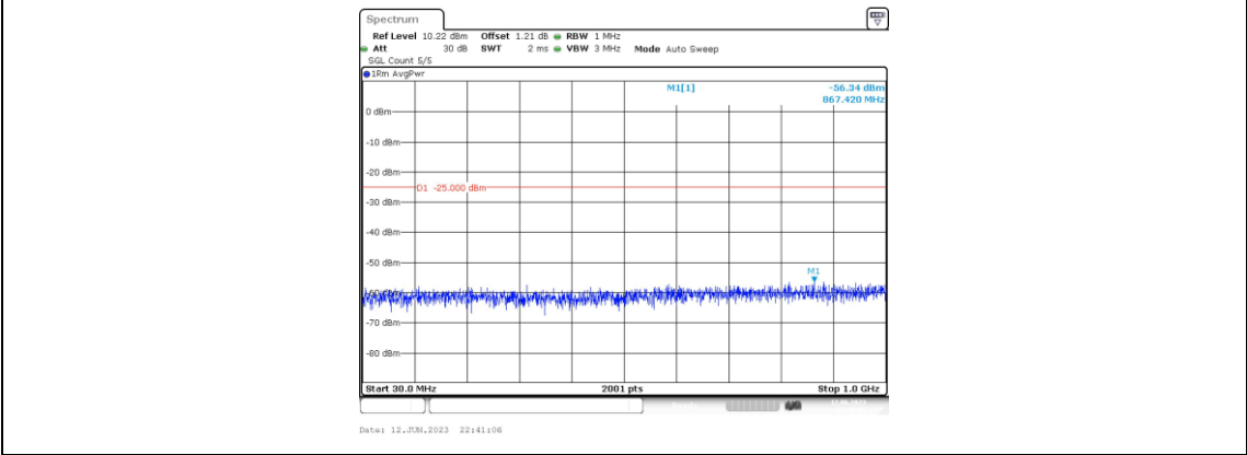
Band7-10MHz-QPSK-20800-1RB#0-Range3:30~1000MHz
