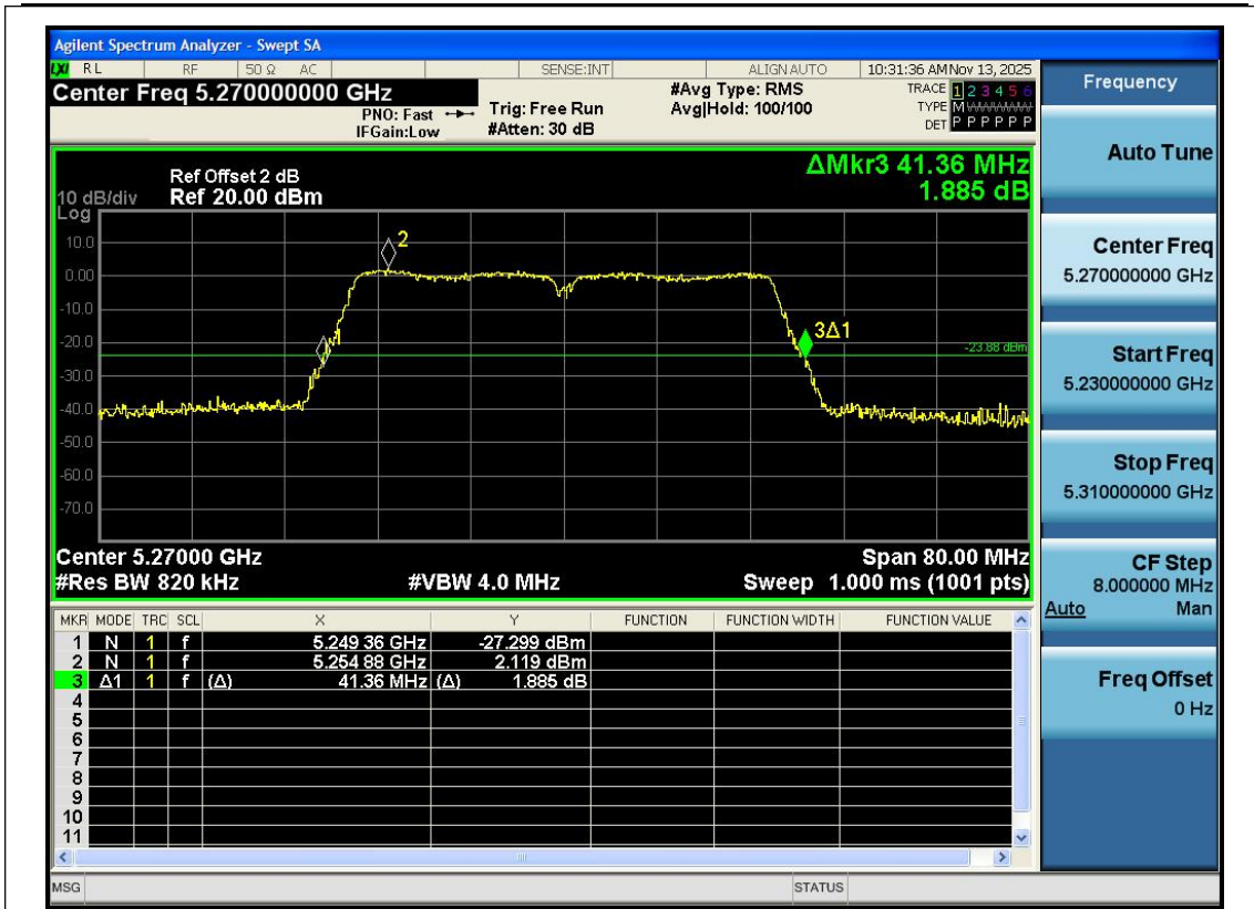
11N40SISO-Ant1-5270
