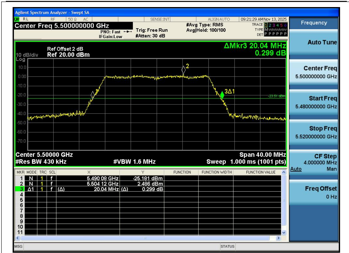
11A-Ant1-5500
