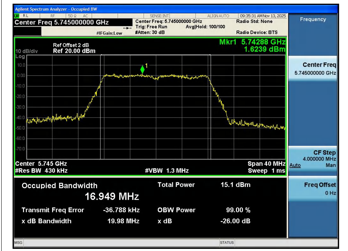
11A-Ant1-5745
