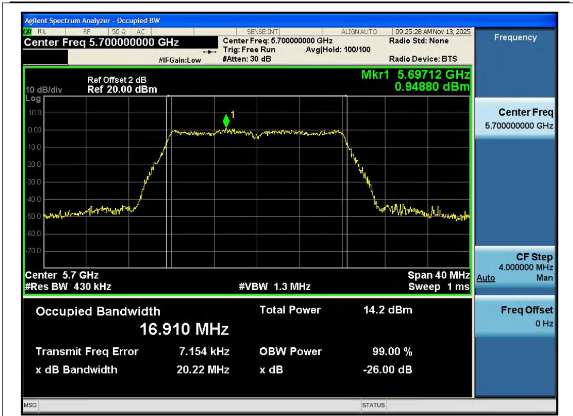
11A-Ant1-5700
