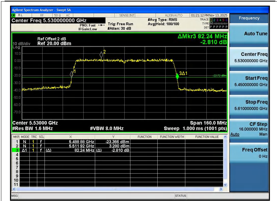
11AC80SISO-Ant1-5530
