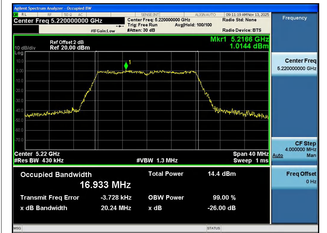
11A-Ant1-5220
