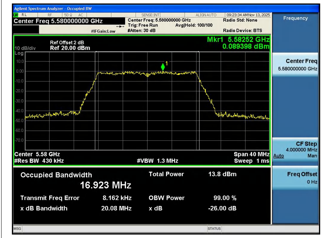
11A-Ant1-5580
