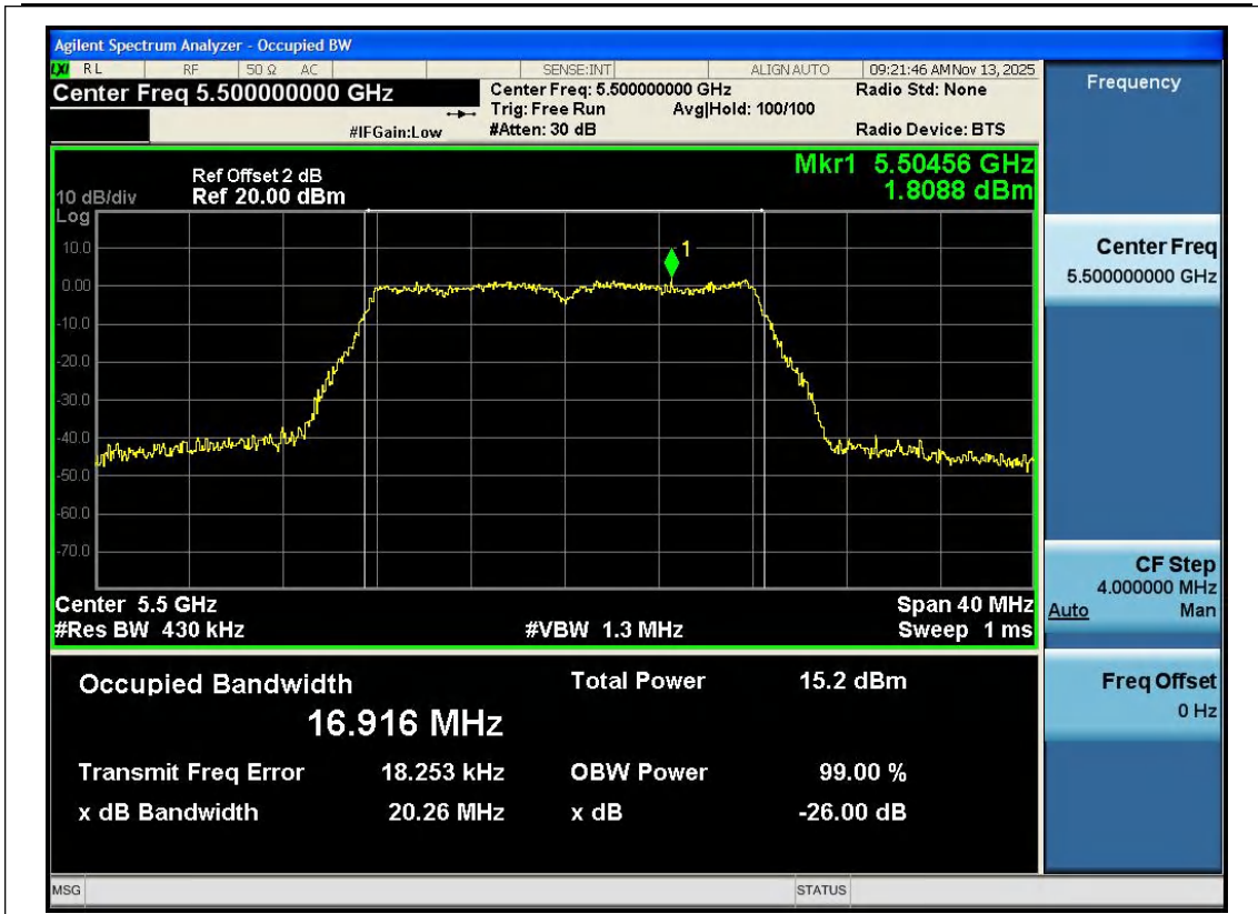
11A-Ant1-5500
