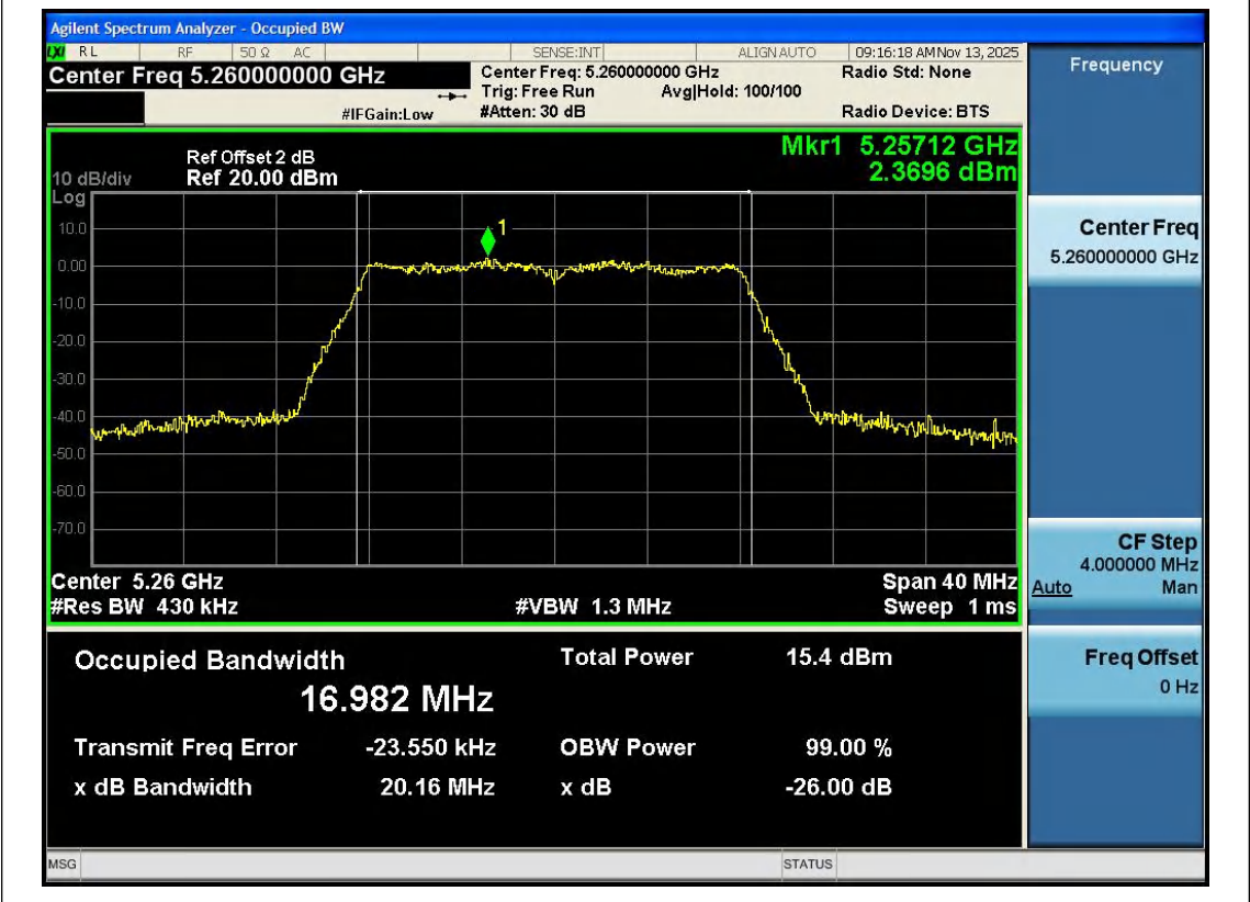
11A-Ant1-5260
