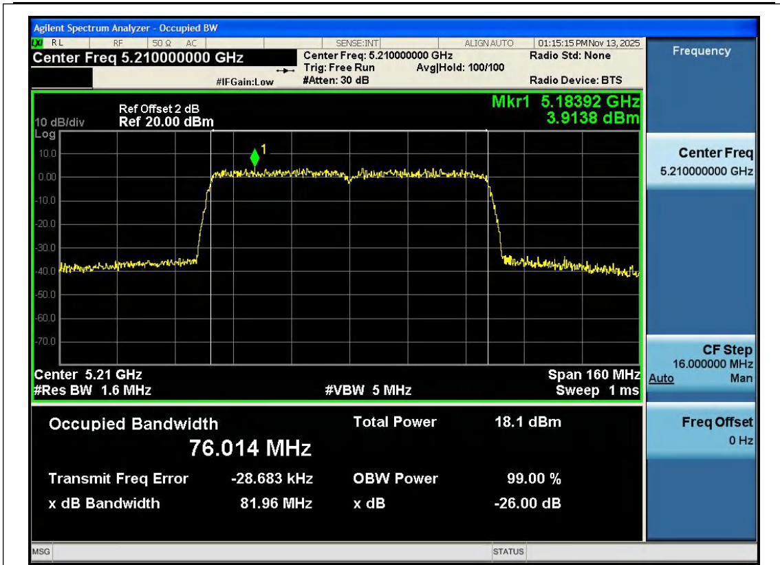
11AC80SISO-Ant1-5210
