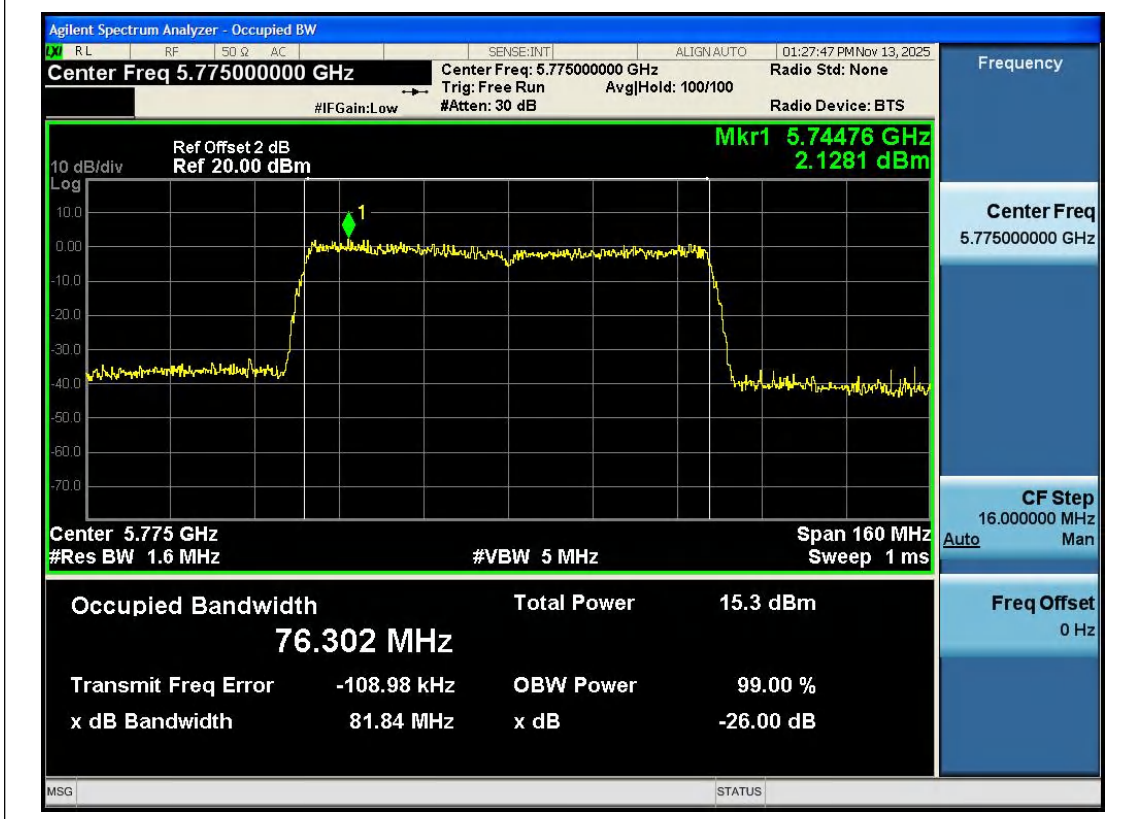
11AC80SISO-Ant1-5775
