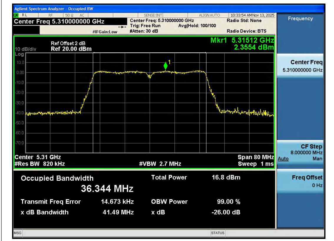
11N40SISO-Ant1-5310
