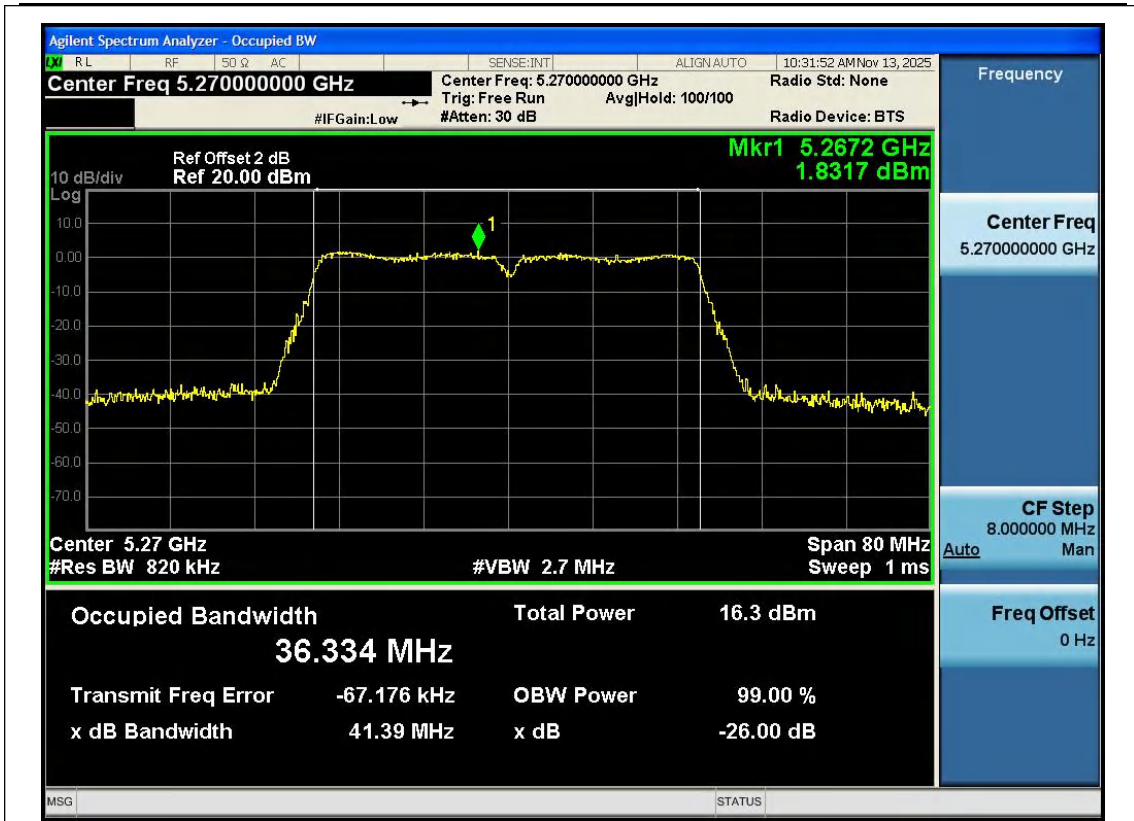
11N40SISO-Ant1-5270
