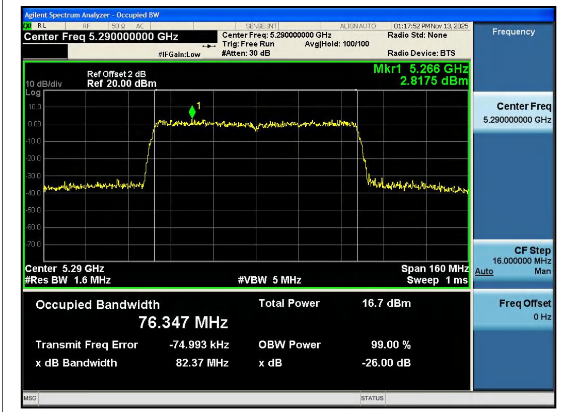
11AC80SISO-Ant1-5290
