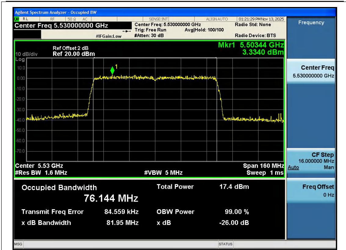
11AC80SISO-Ant1-5530
