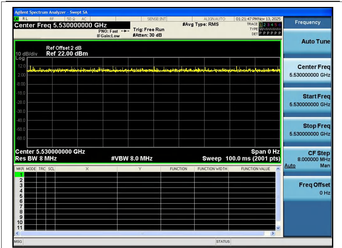
NTNV-11AC80SISO-Ant1-5530
