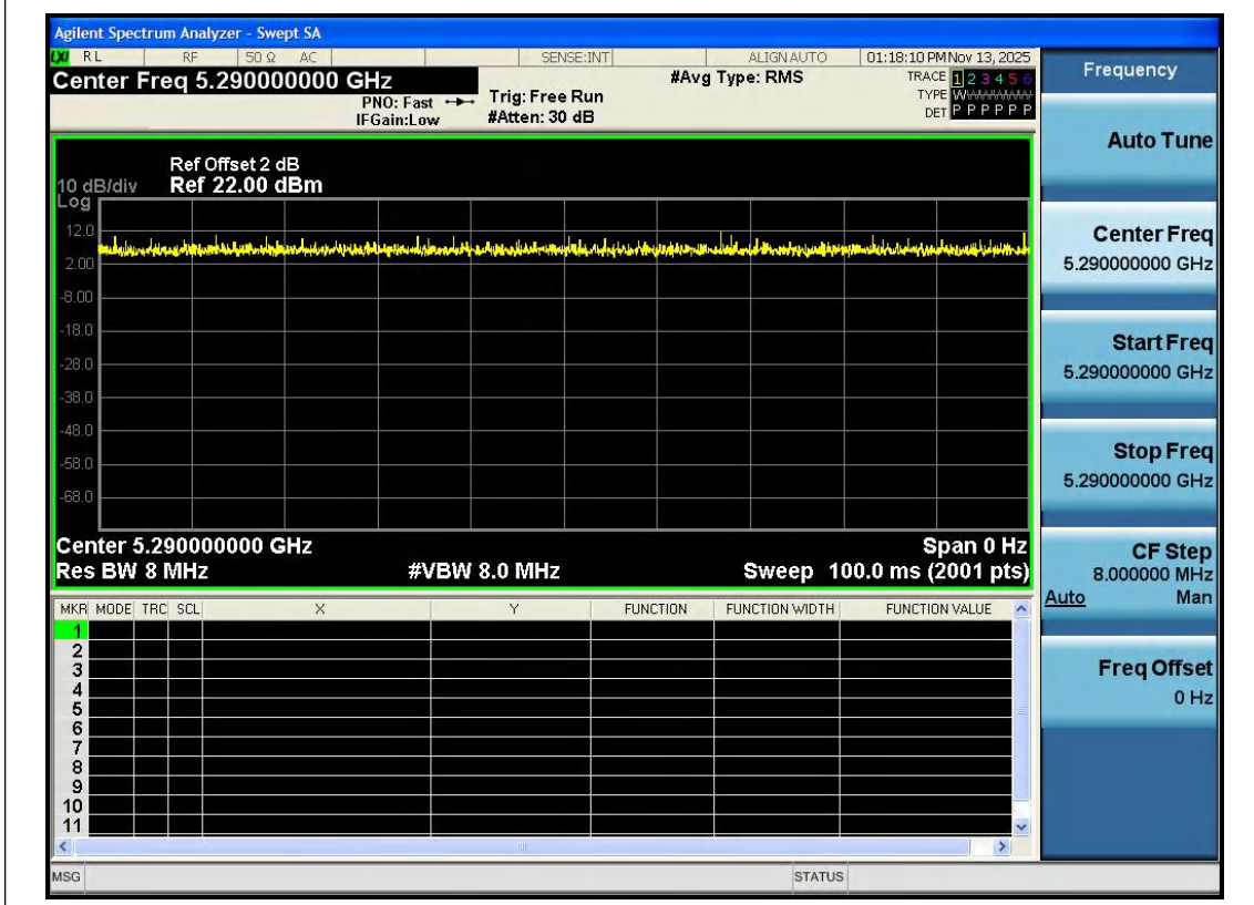
NTNV-11AC80SISO-Ant1-5290
