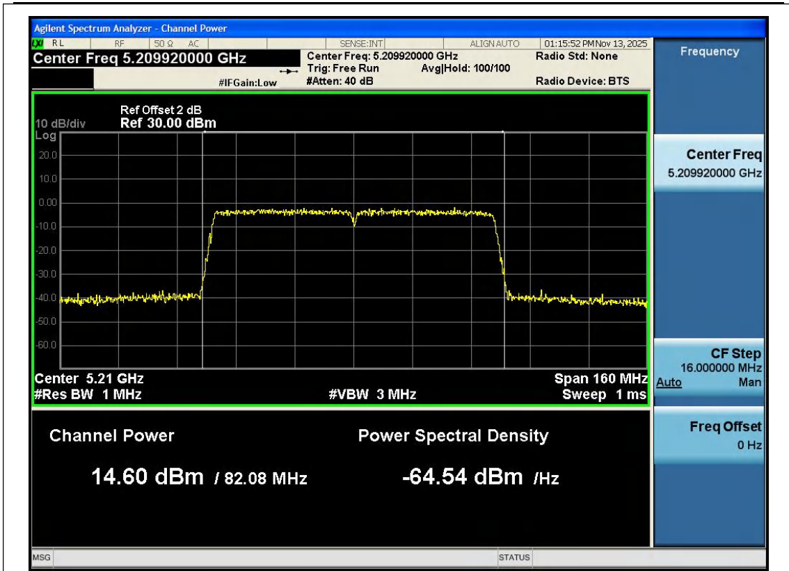
11AC80SISO-Ant1-5210-PASS
