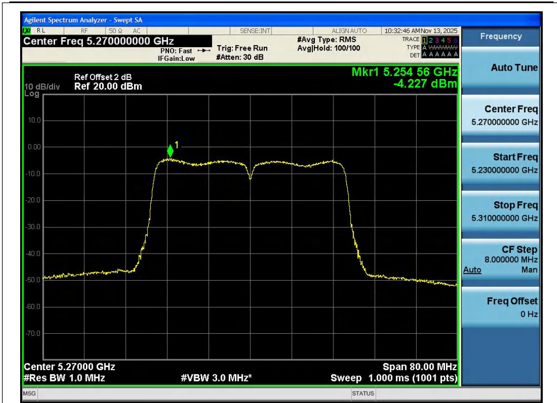
11N40SISO-Ant1-5270-PASS
