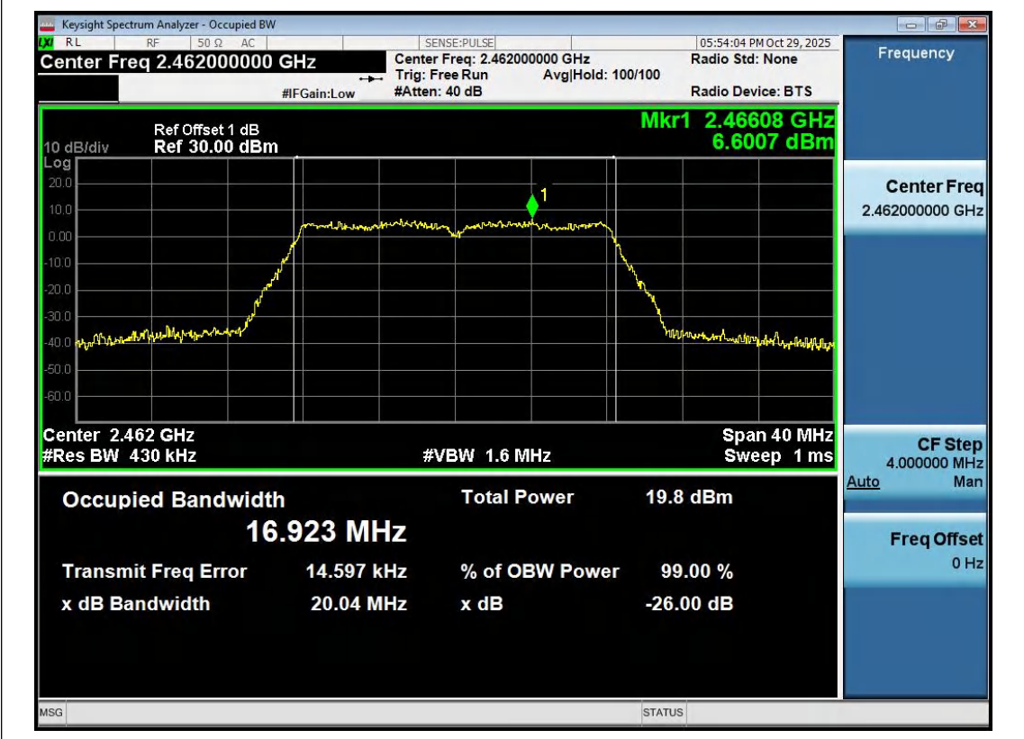
11G-Ant1-2462
