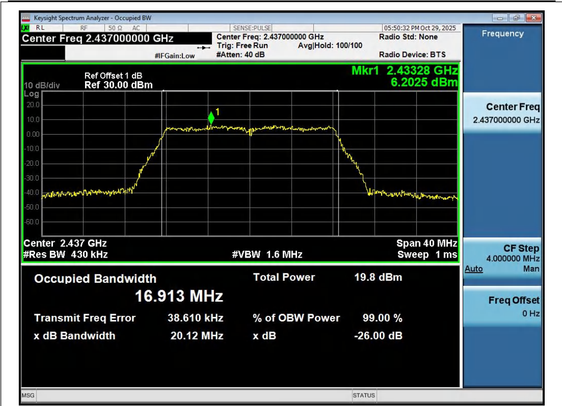
11G-Ant1-2437
