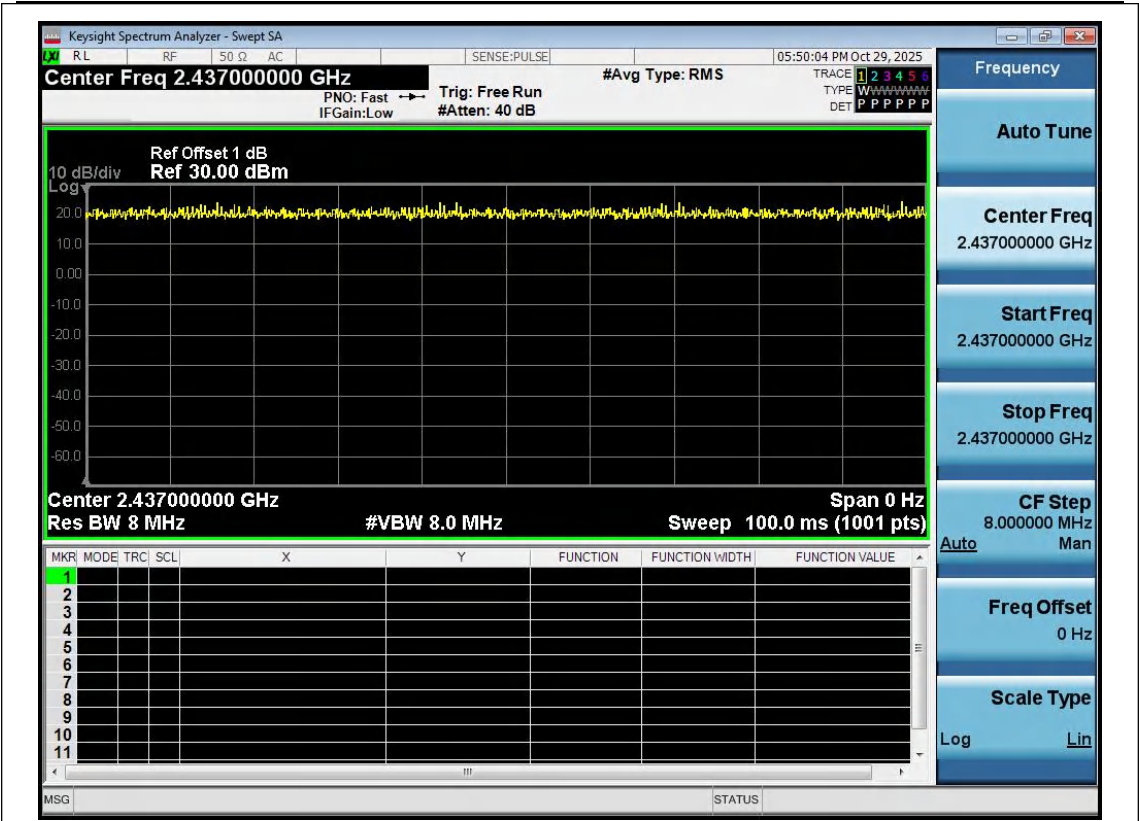
NTNV-11G-Ant1-2437
