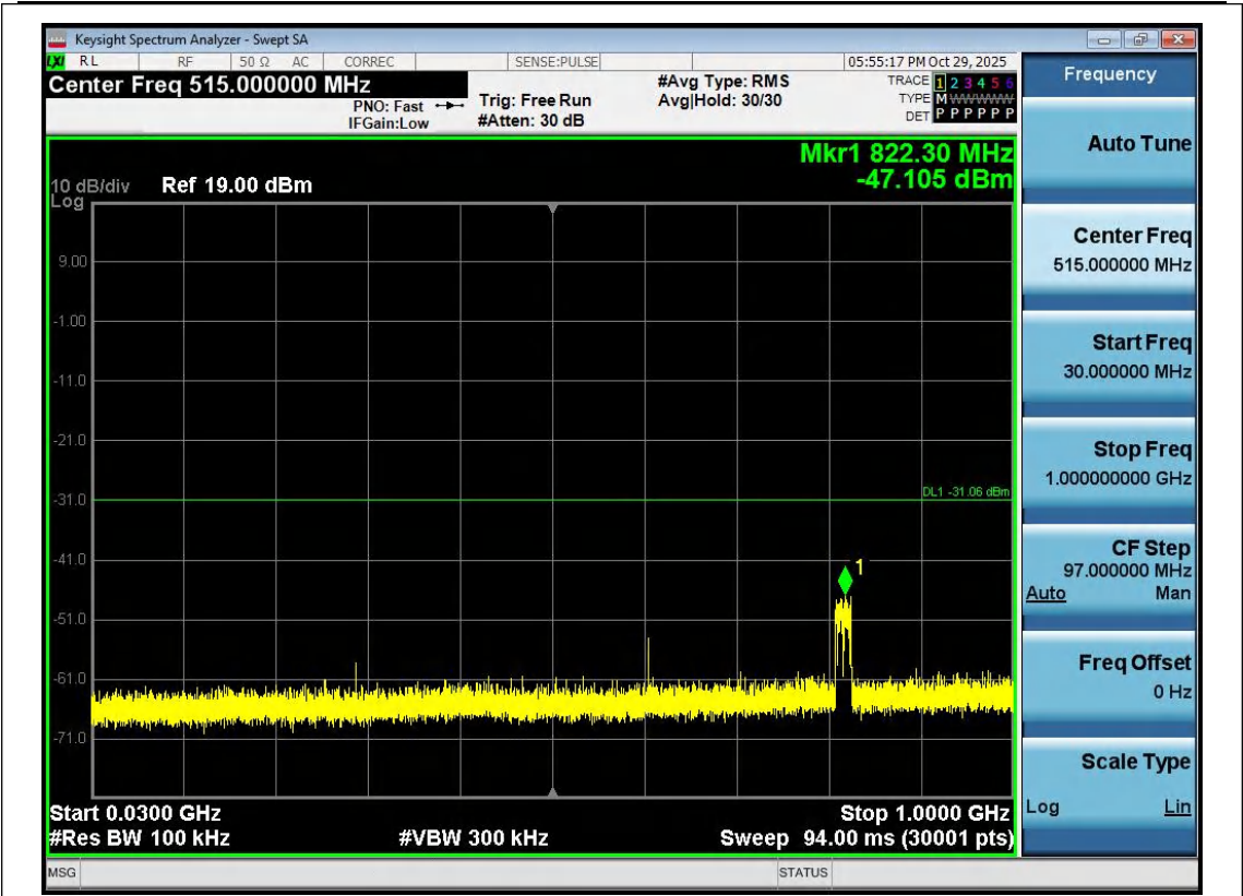
11G-Ant1-2462-30~1000-PASS
