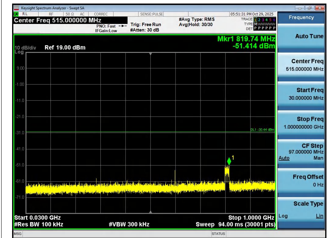
11G-Ant1-2437-30~1000-PASS
