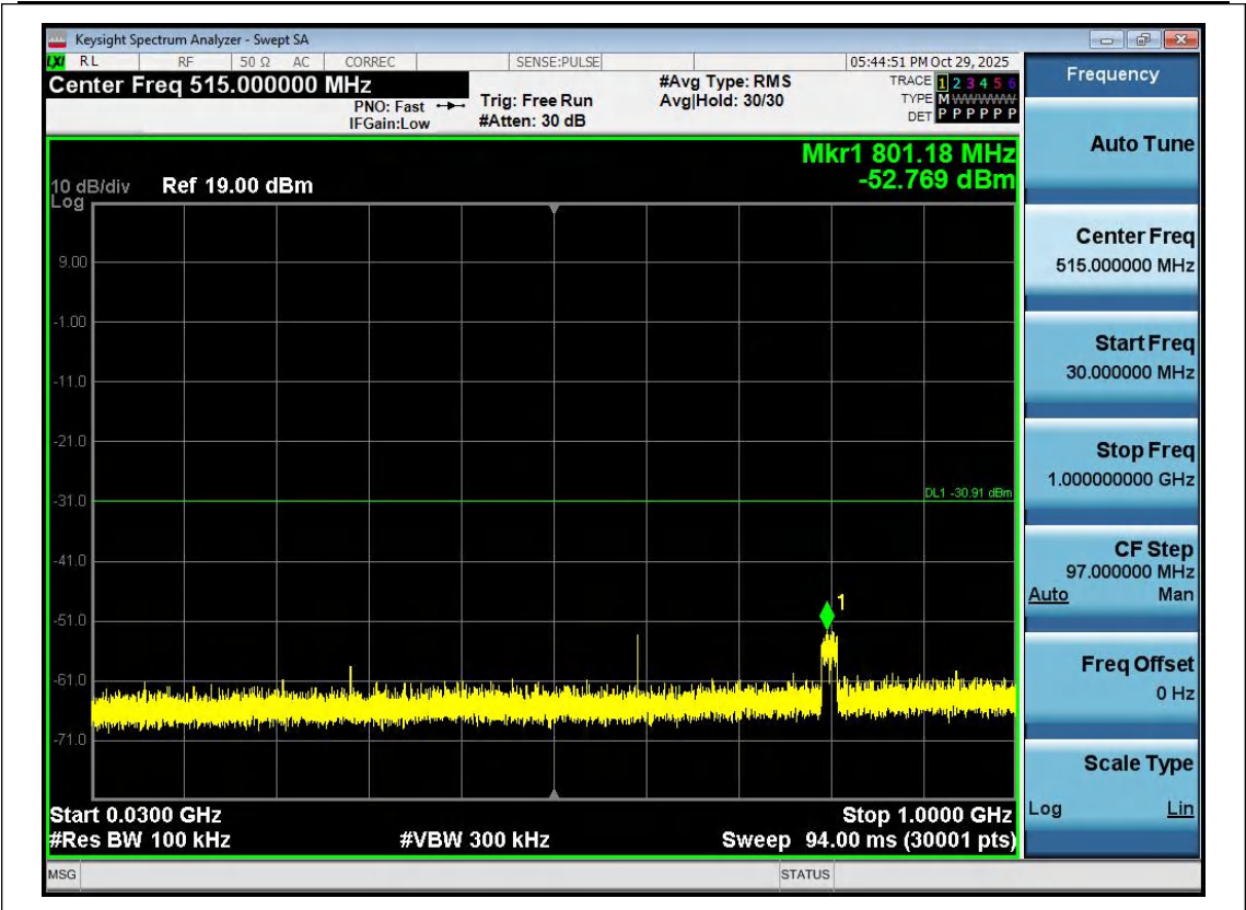
11G-Ant1-2412-30~1000-PASS
