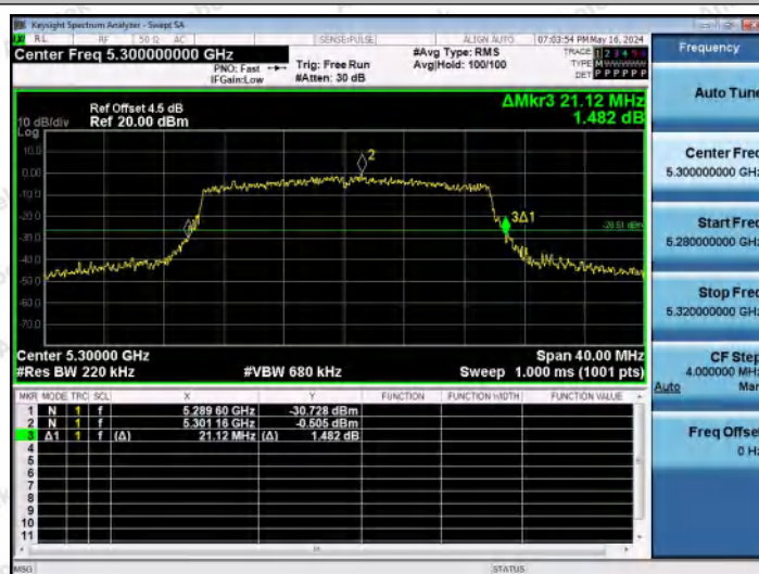
11AX20MIMO-Ant2-5300
