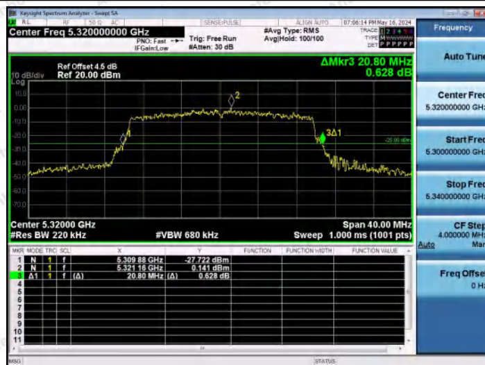
11AX20MIMO-Ant2-5320
