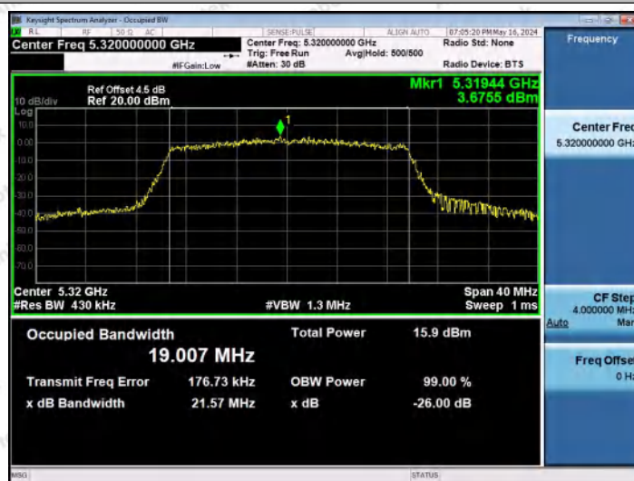
11AX20MIMO-Ant1-5320
