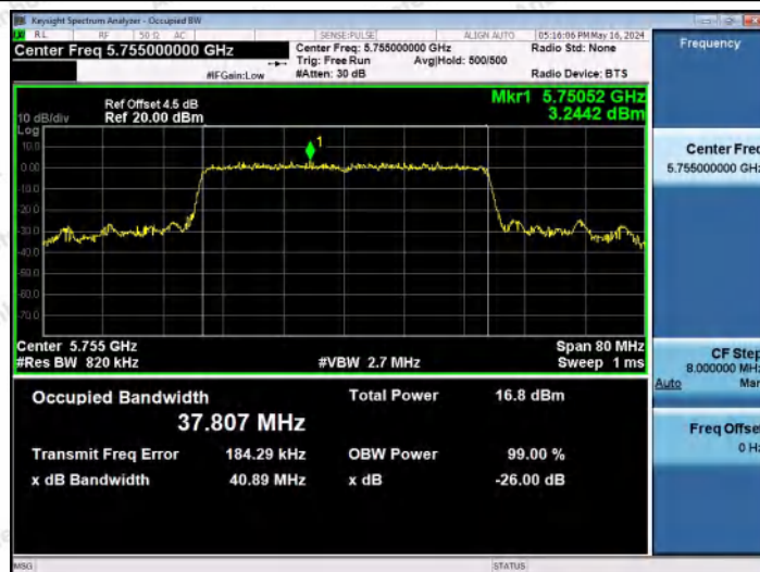
11AX40MIMO-Ant1-5755
