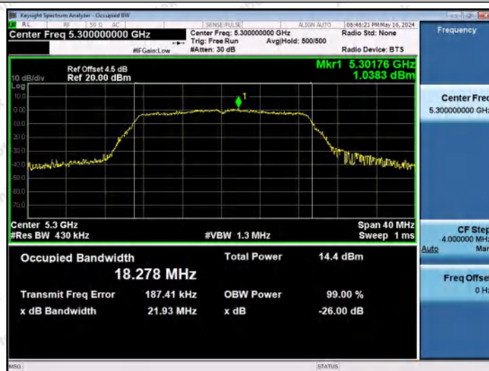
11AC20MIMO-Ant1-5300
