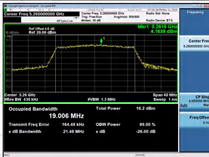
11AX20MIMO-Ant1-5260
