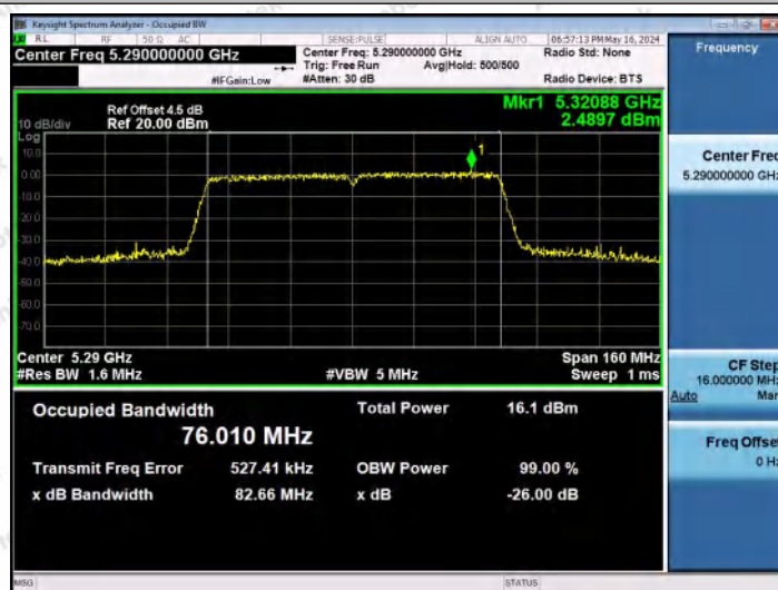
11AC80MIMO-Ant1-5290
