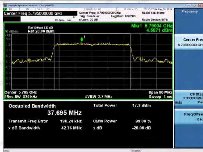
11AX40MIMO-Ant2-5795
