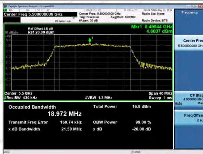
11AX20MIMO-Ant2-5500
