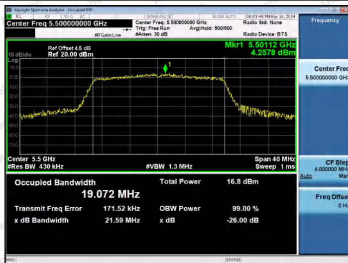
11AX20MIMO-Ant1-5500
