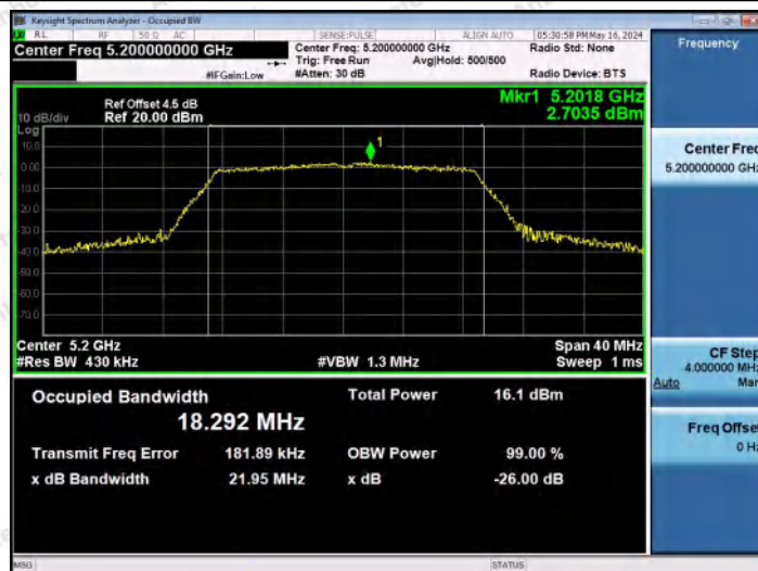
11N20MIMO-Ant2-5200
