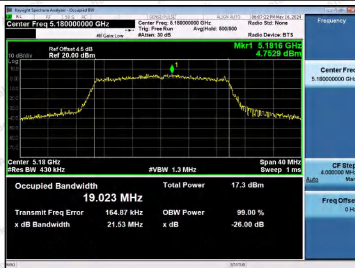
11AX20MIMO-Ant1-5180
