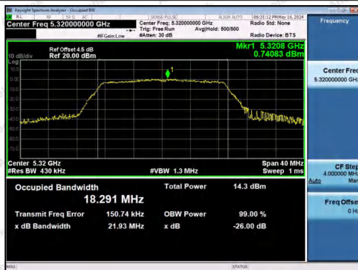
11N20MIMO-Ant1-5320
