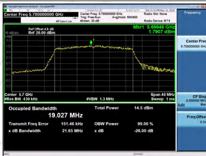
11AX20MIMO-Ant1-5700
