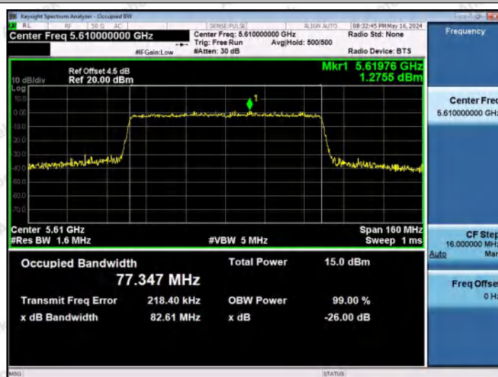
11AX80MIMO-Ant1-5610
