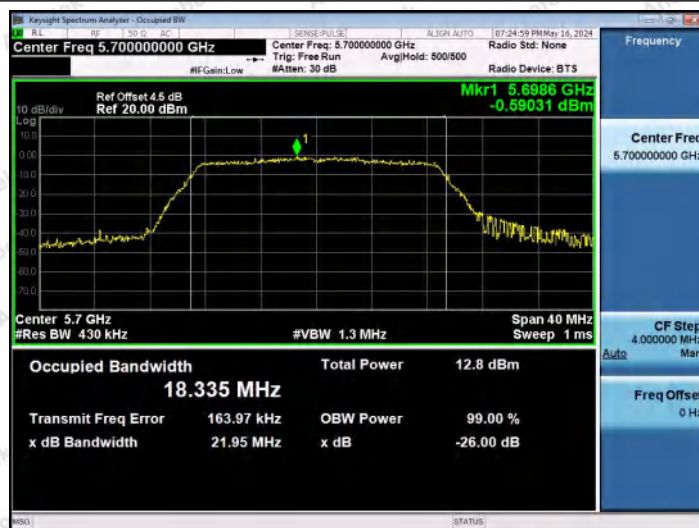
11N20MIMO-Ant1-5700
