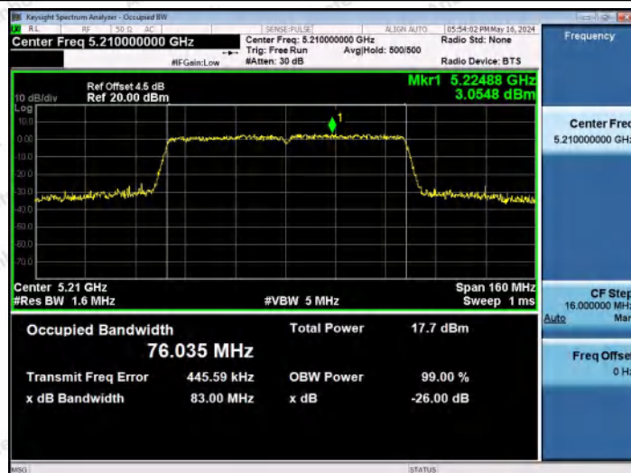
11AC80MIMO-Ant1-5210
