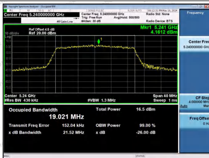
11AX20MIMO-Ant1-5240
