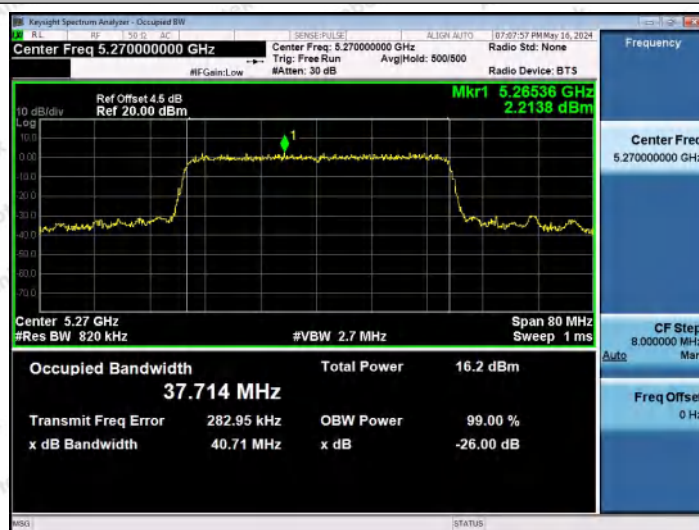
11AX40MIMO-Ant1-5270
