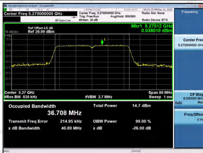
11AC40MIMO-Ant1-5270
