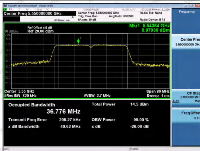
11N40MIMO-Ant1-5550
