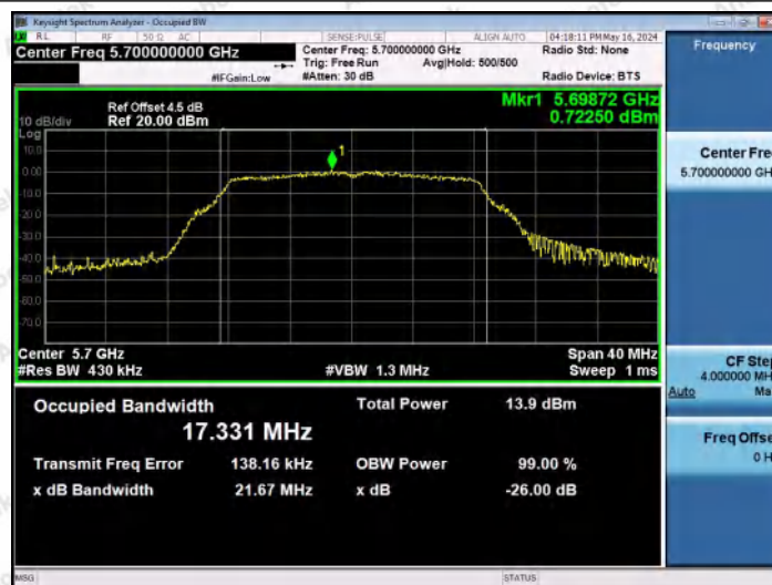
11A-Ant1-5700
