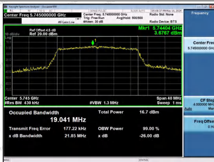
11AX20MIMO-Ant2-5745
