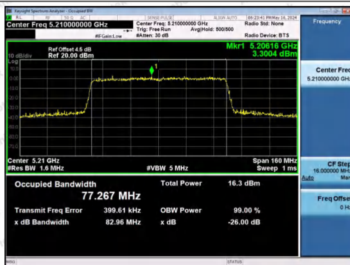
11AX80MIMO-Ant2-5210
