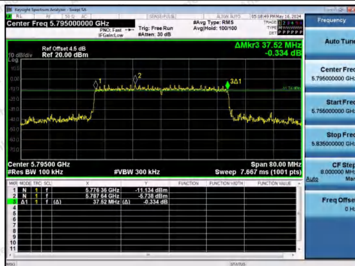
11AX40MIMO-Ant1-5795-PASS
