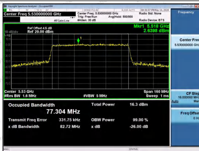
11AX80MIMO-Ant1-5530
