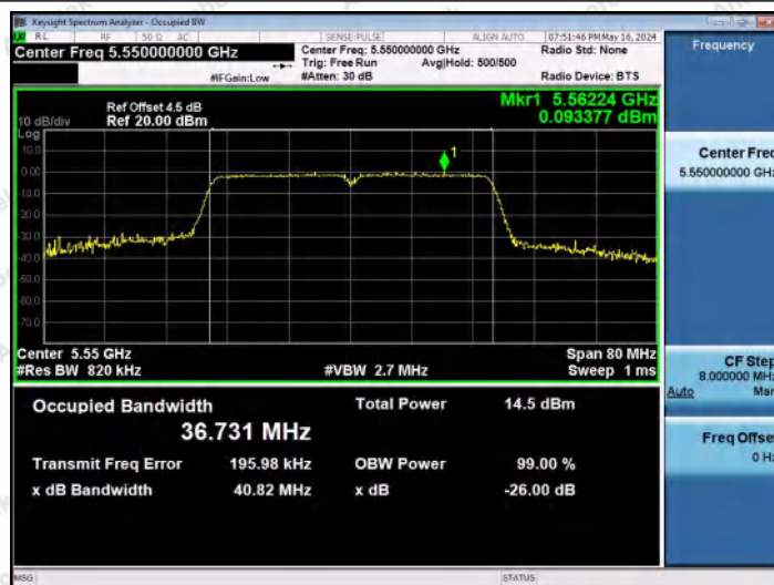
11AC40MIMO-Ant1-5550
