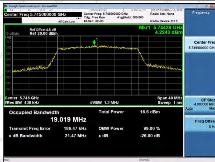
11AX20MIMO-Ant1-5745
