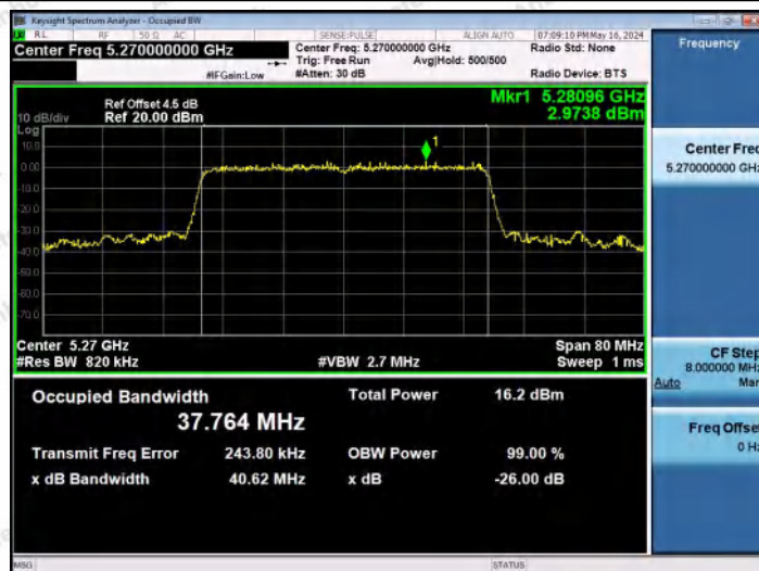
11AX40MIMO-Ant2-5270
