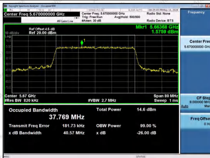
11AX40MIMO-Ant1-5670
