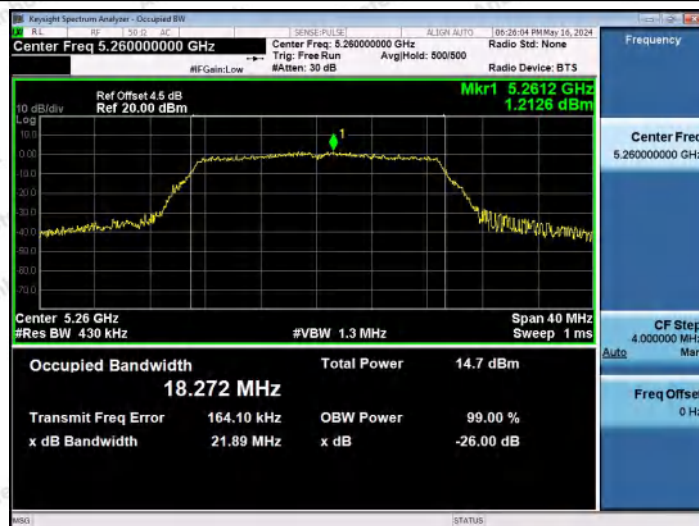
11N20MIMO-Ant1-5260
