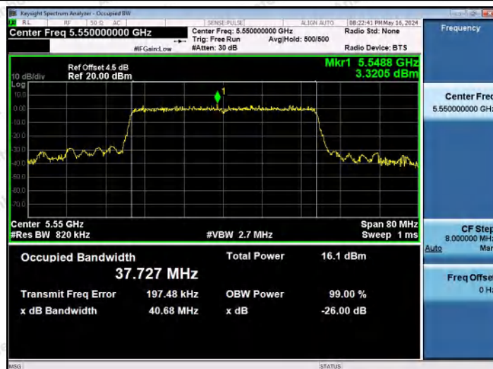
11AX40MIMO-Ant2-5550
