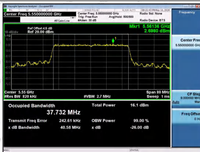
11AX40MIMO-Ant1-5550
