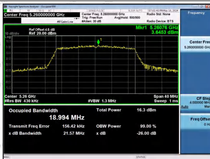
11AX20MIMO-Ant2-5260
