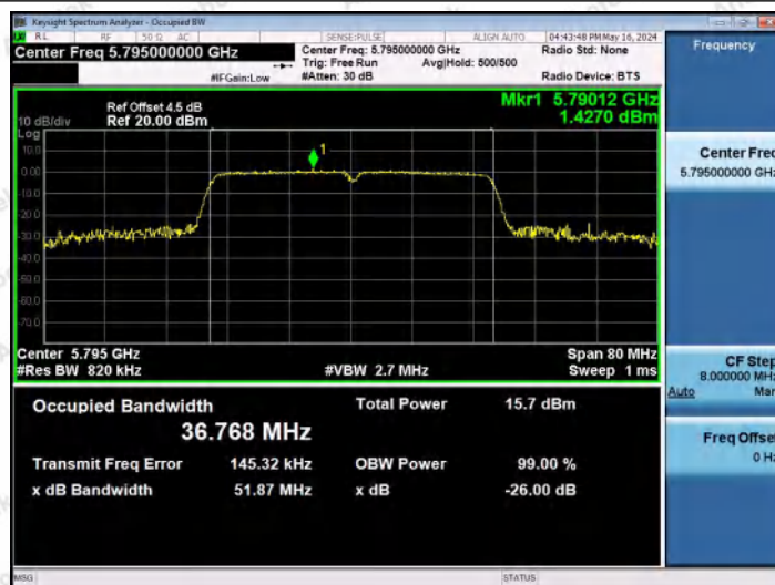
11N40MIMO-Ant1-5795
