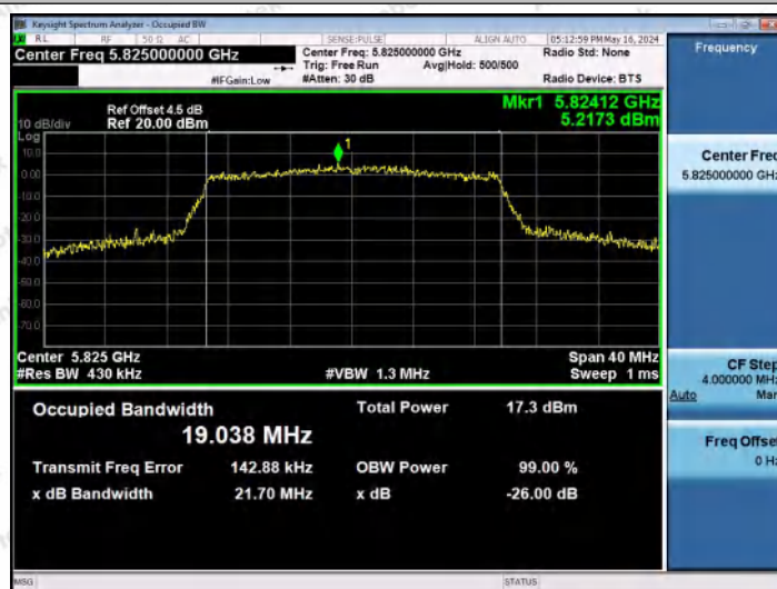
11AX20MIMO-Ant1-5825
