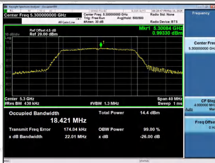
11N20MIMO-Ant1-5300
