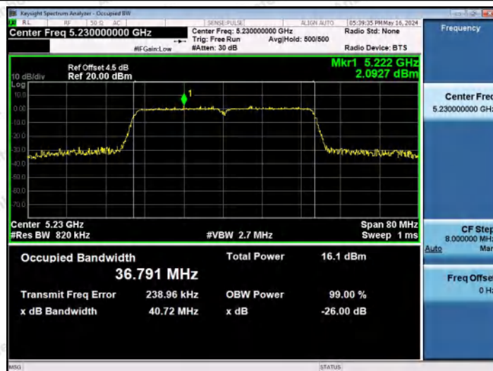
11N40MIMO-Ant2-5230
