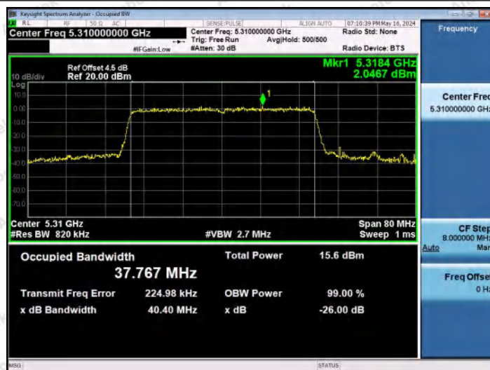
11AX40MIMO-Ant1-5310
