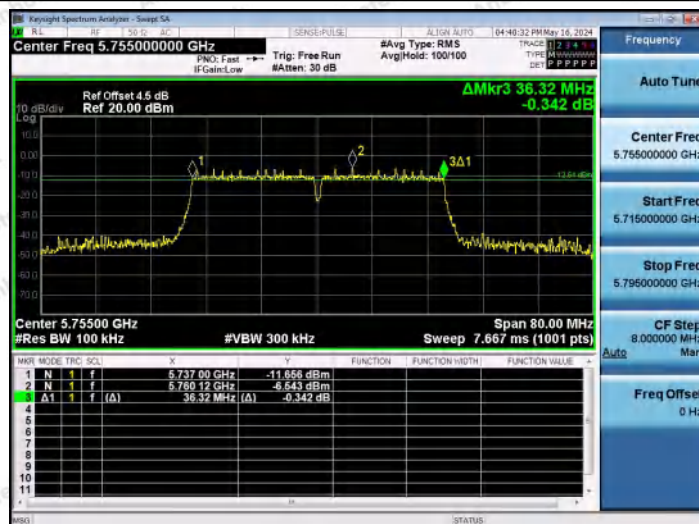
11N40MIMO-Ant1-5755-PASS
