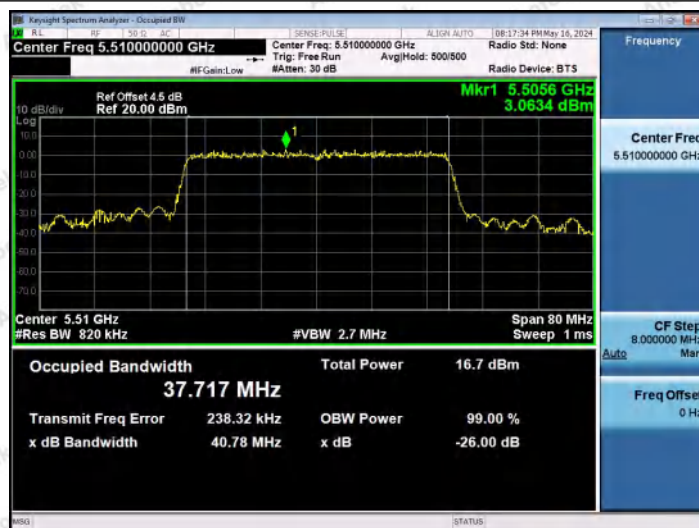
11AX40MIMO-Ant2-5510
