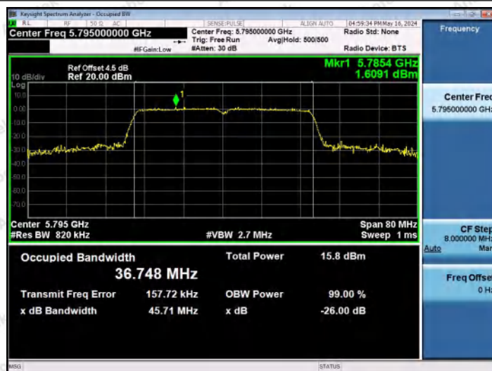
11AC40MIMO-Ant1-5795
