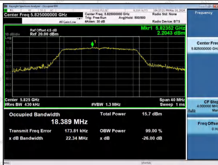
11N20MIMO-Ant1-5825
