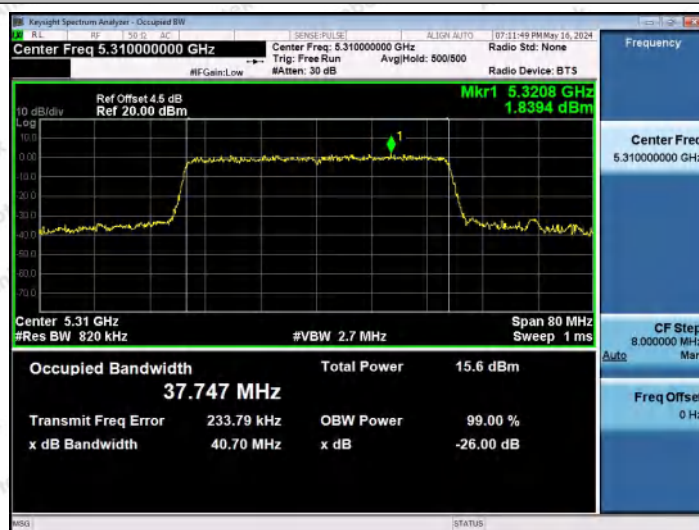
11AX40MIMO-Ant2-5310
