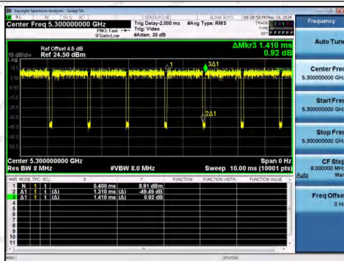
NTNV-11N20MIMO-Ant1-5300
