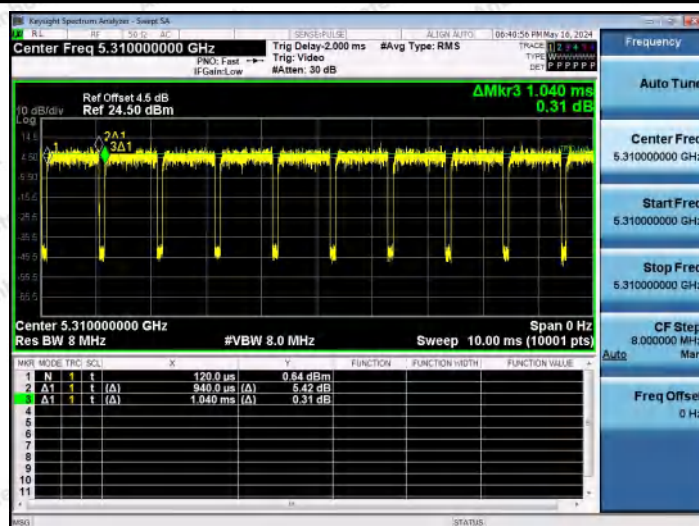
NTNV-11N40MIMO-Ant1-5310
