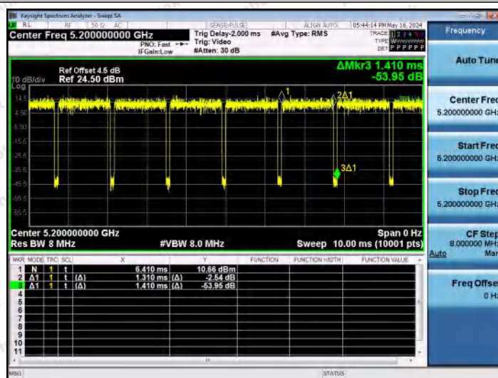
NTNV-11AC20MIMO-Ant1-5200
