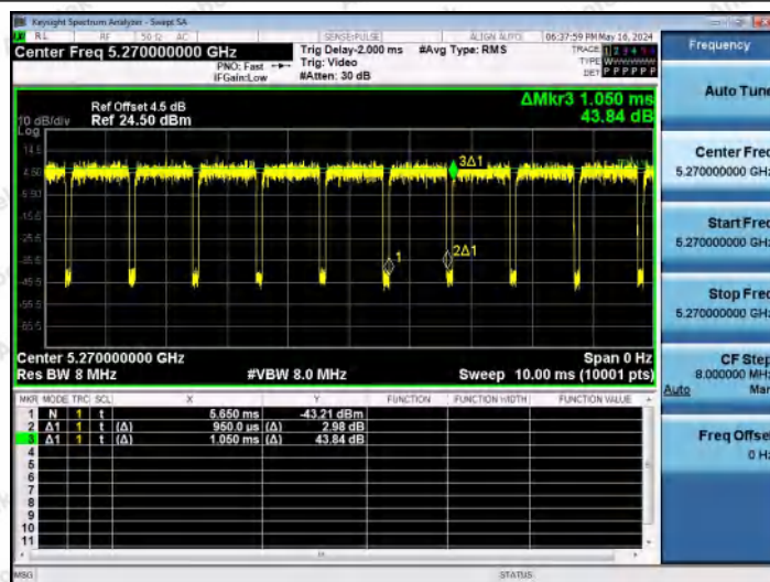
NTNV-11N40MIMO-Ant1-5270
