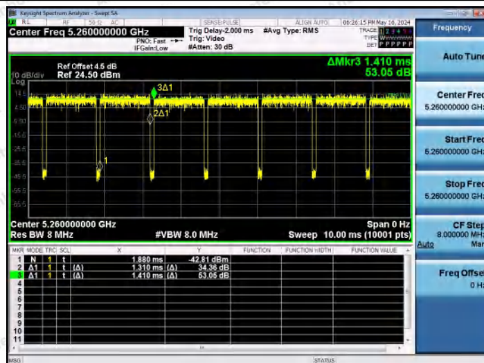
NTNV-11N20MIMO-Ant1-5260
