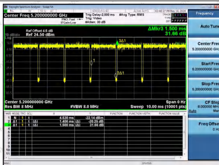
NTNV-11A-Ant1-5200
