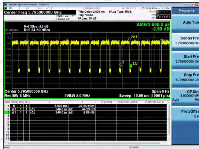
NTNV-11AX40MIMO-Ant2-5795
