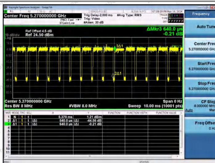
NTNV-11AX40MIMO-Ant1-5270
