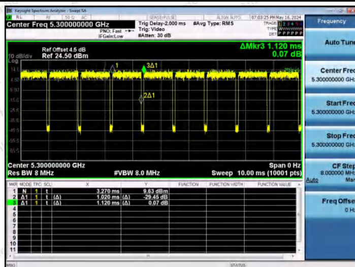
NTNV-11AX20MIMO-Ant1-5300
