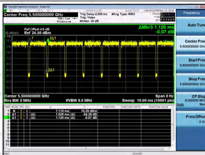
NTNV-11AX20MIMO-Ant1-5500
