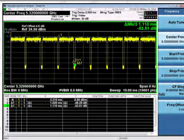
NTNV-11AX20MIMO-Ant1-5320
