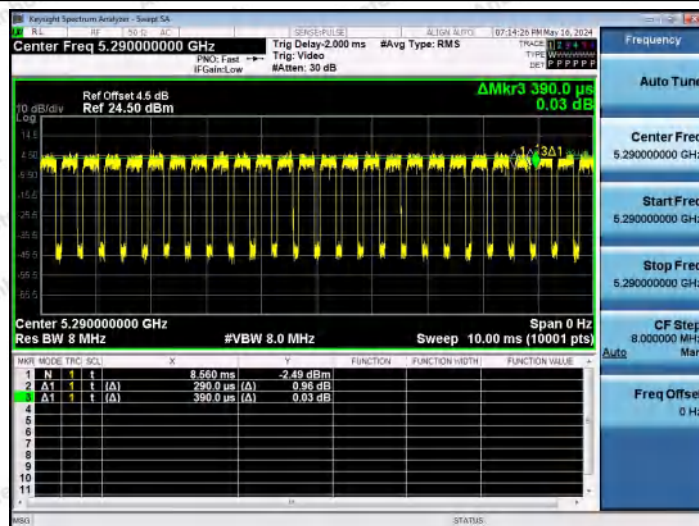
NTNV-11AX80MIMO-Ant1-5290
