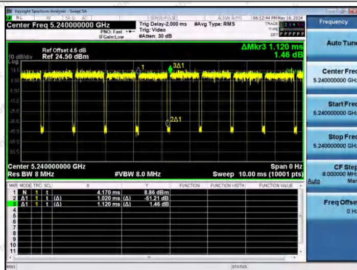
NTNV-11AX20MIMO-Ant1-5240
