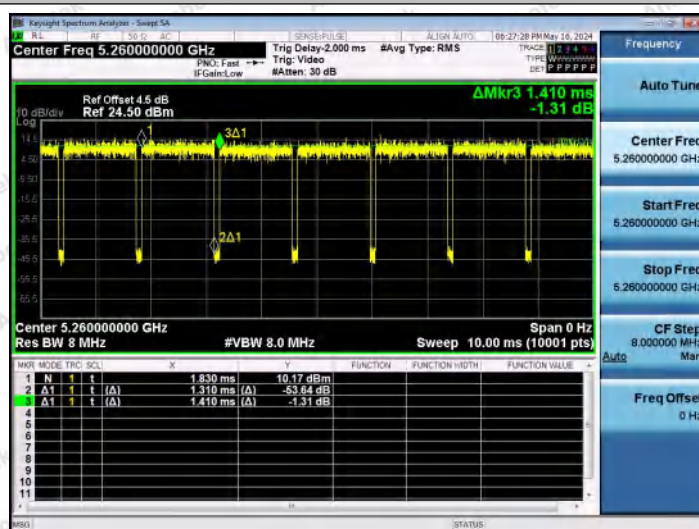
NTNV-11N20MIMO-Ant2-5260
