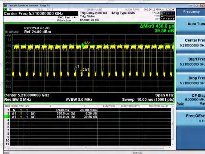
NTNV-11AC80MIMO-Ant1-5210
