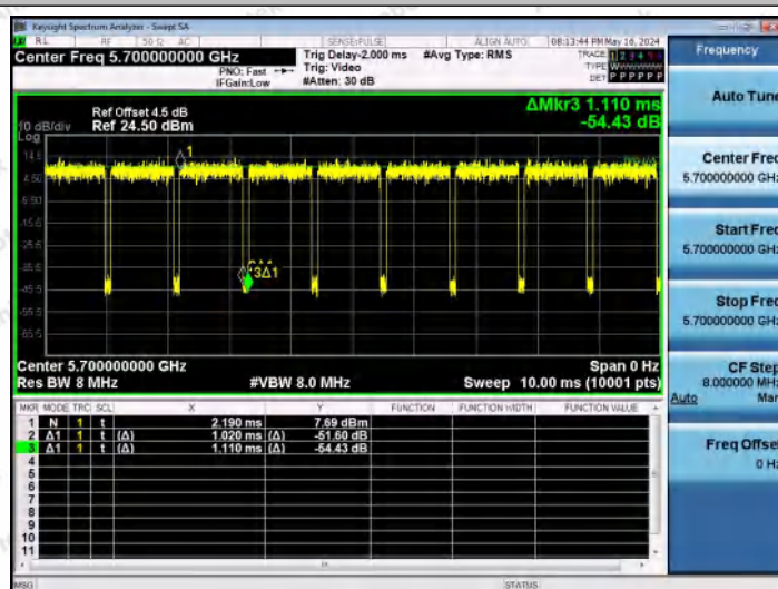
NTNV-11AX20MIMO-Ant1-5700
