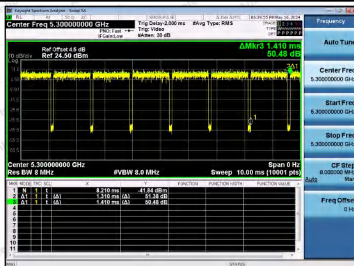
NTNV-11N20MIMO-Ant2-5300
