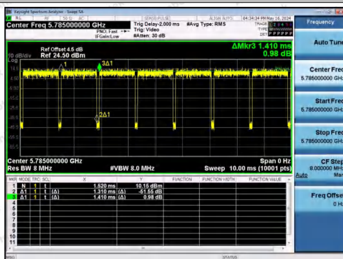
NTNV-11N20MIMO-Ant1-5785
