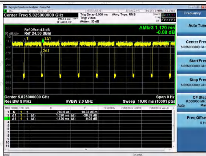
NTNV-11AX20MIMO-Ant1-5825
