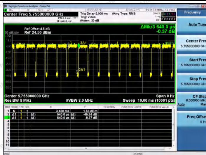
NTNV-11AX40MIMO-Ant1-5755
