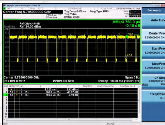
NTNV-11AC40MIMO-Ant1-5795
