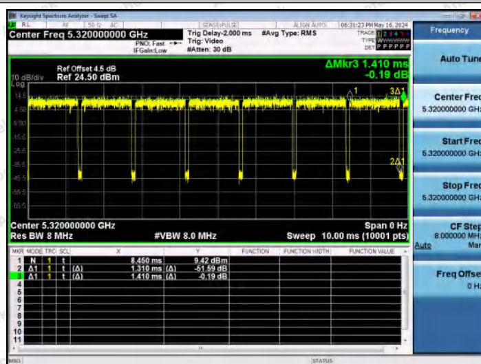
NTNV-11N20MIMO-Ant1-5320
