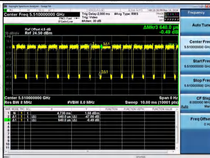
NTNV-11AX40MIMO-Ant1-5510
