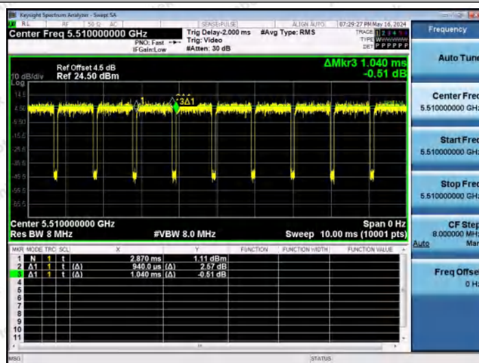
NTNV-11N40MIMO-Ant1-5510
