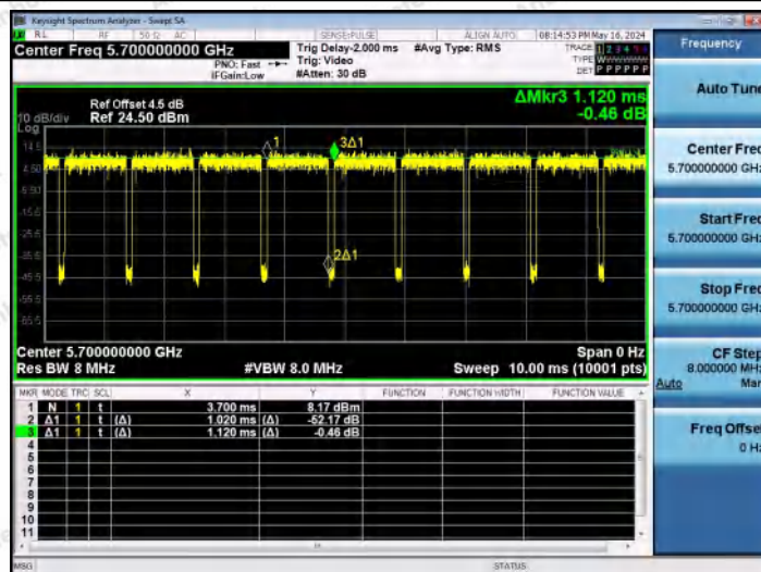
NTNV-11AX20MIMO-Ant2-5700
