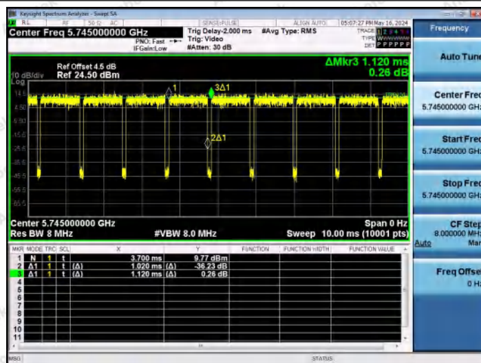
NTNV-11AX20MIMO-Ant1-5745
