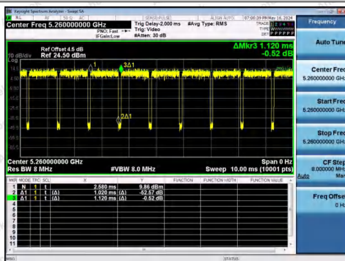
NTNV-11AX20MIMO-Ant1-5260
