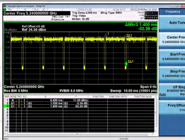
NTNV-11N20MIMO-Ant1-5240
