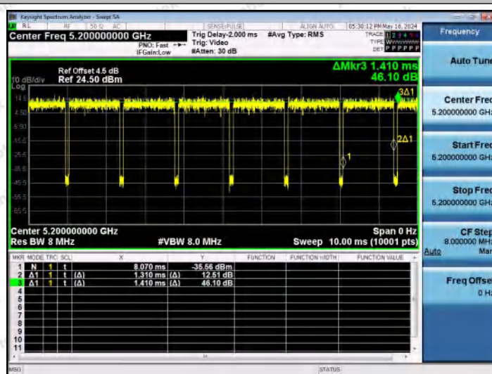
NTVN-11N20MIMO-Ant1-5200
