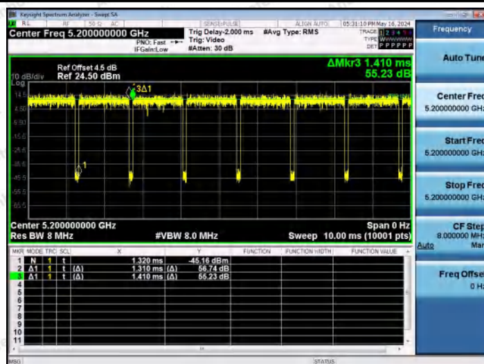
NTNV-11N20MIMO-Ant2-5200
