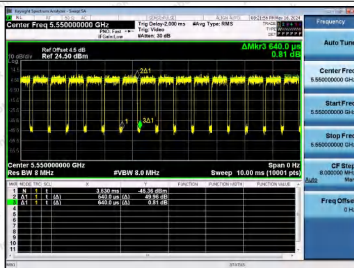
NTNV-11AX40MIMO-Ant1-5550
