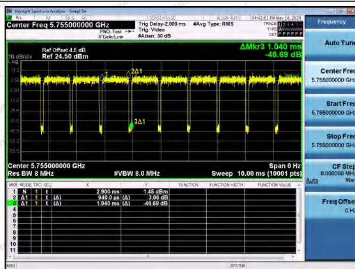
NTNV-11N40MIMO-Ant1-5755
