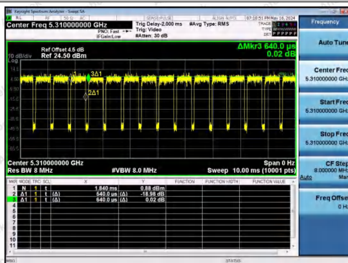
NTNV-11AX40MIMO-Ant1-5310
