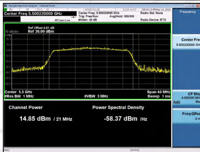
11AX20MIMO-Ant1-5500-PASS
