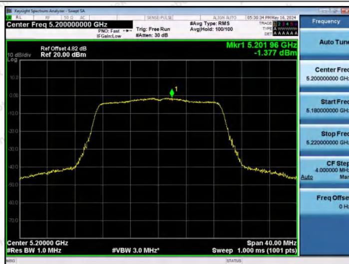
11N20MIMO-Ant1-5200-PASS
